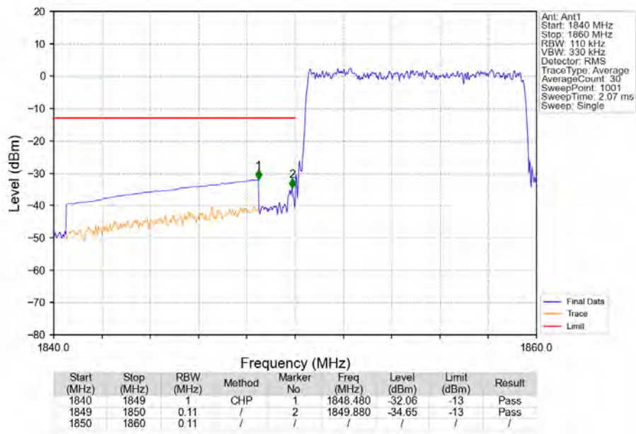
Band25 10MHz 16QAM LCH 1855MHz RB 50 0 NTV
