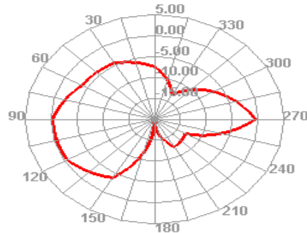
2450.000MHz E1
