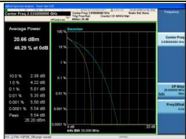
Band 7 CH21100(2535MHz) QPSK-20MHz
