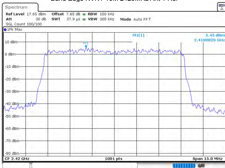
Band Edge NVNT 10M 2420MHz Ant 1 Ref
