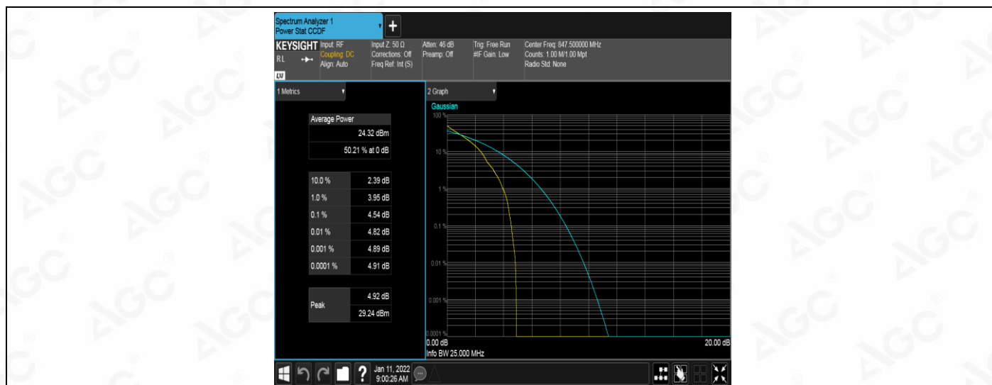
Band5-3MHz-QPSK-20635-15RB#0
