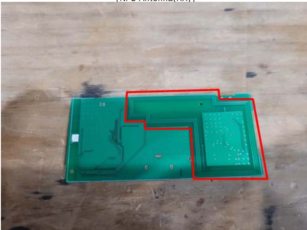
{ NFC Antenna(RX) }
