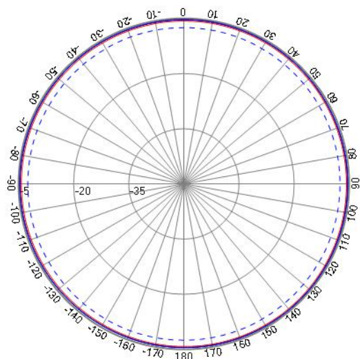
XY-PLANE
