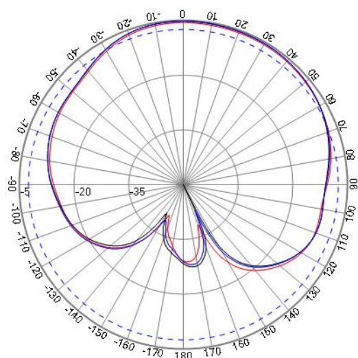
XZ-PLANE
