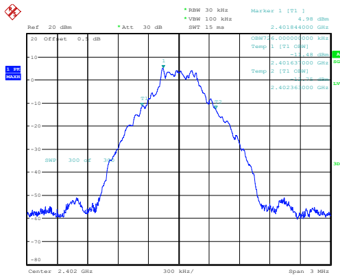
GFSK_Low 0.726MHz
