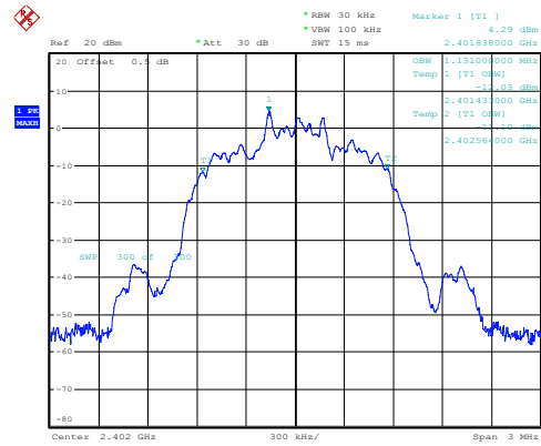
\pi/4 -DQPSK_Low 1.131MHz
