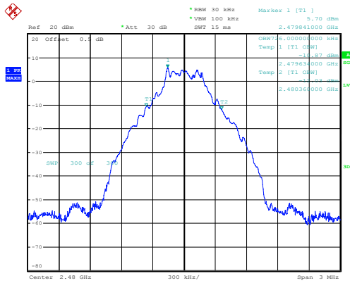
GFSK_High 0.726MHz
