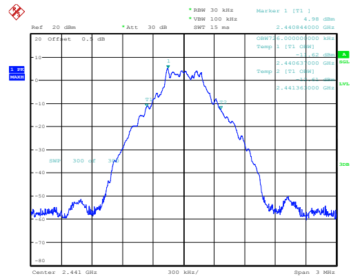
GFSK_Middle 0.726MHz
