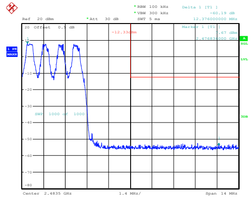
GFSK_Hopping_Upper 60.19dB
