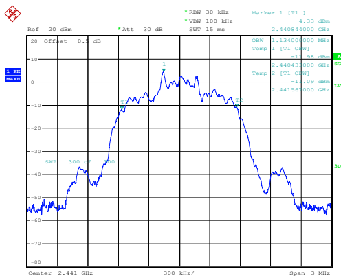
\pi/4 -DQPSK_Middle 1.134MHz
