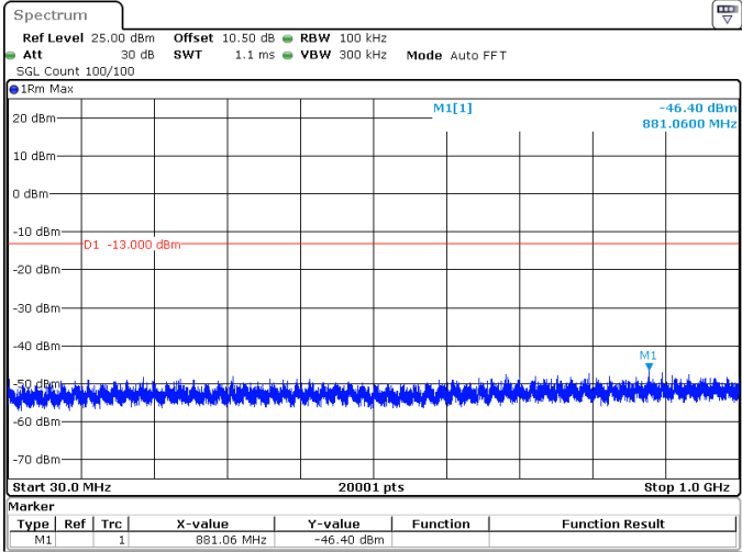
90MHz_30kHz_3745MHz_DFT-s-OFDM QPSK_RB243@0 -46.40 dBm
