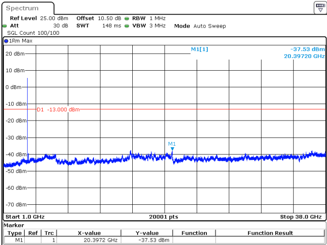
90MHz_30kHz_3745MHz_DFT-s-OFDM QPSK_RB1@0 -37.53 dBm
