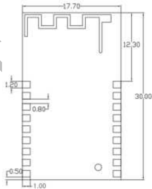
Fig 3 BL3383-P Module Dimensions
