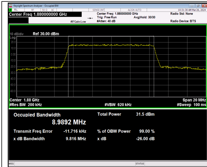
Band2-10MHz-QPSK-18900-50RB#0-PASS
