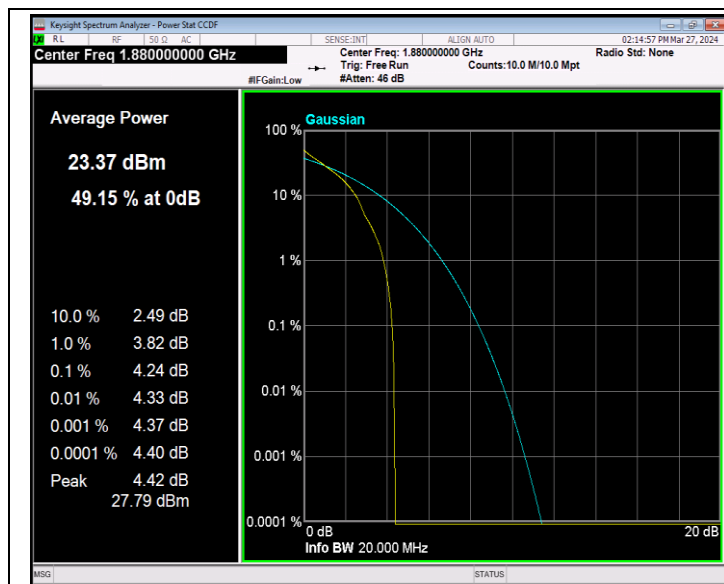
Band2-20MHz-QPSK-18900-1RB#0-PASS
