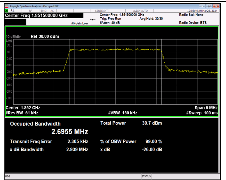
Band2-3MHz-QPSK-18615-15RB#0-PASS
