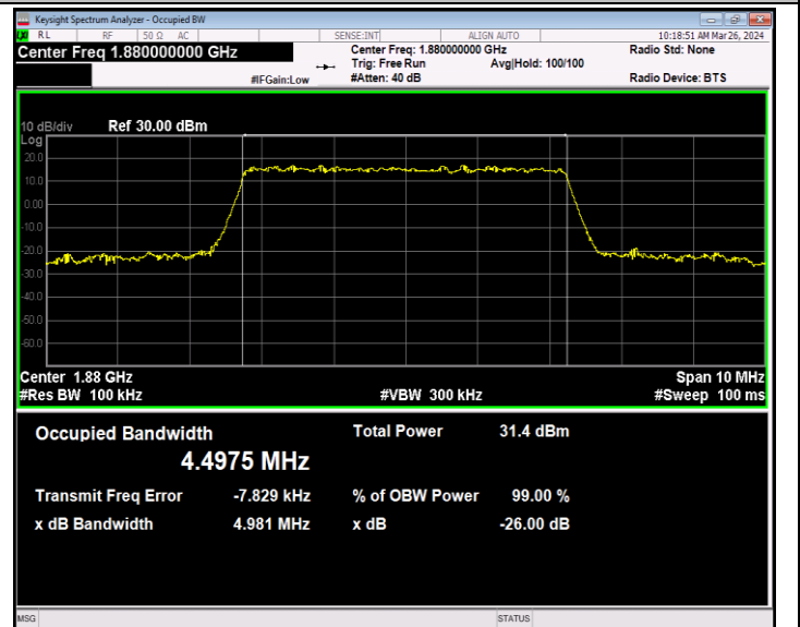
Band2-5MHz-QPSK-18900-25RB#0-PASS
