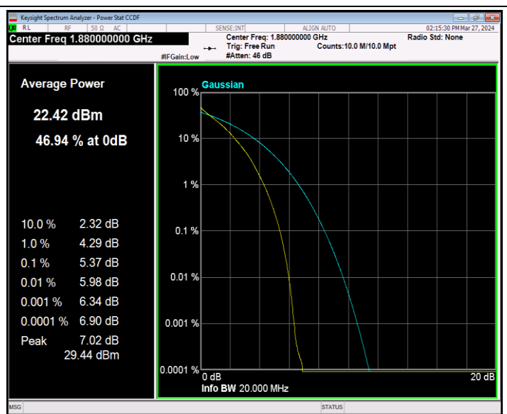
Band2-20MHz-QPSK-18900-100RB#0-PASS
