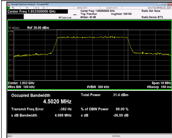
Band2-5MHz-QPSK-18625-25RB#0-PASS
