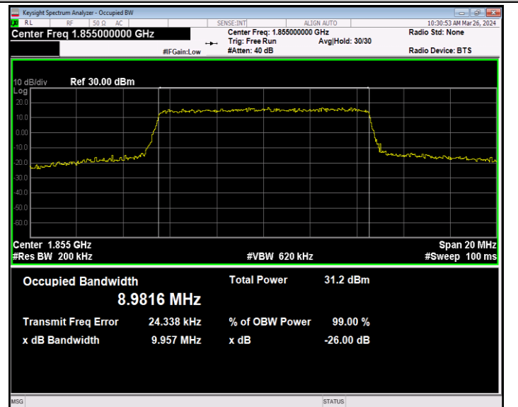
Band2-10MHz-QPSK-18650-50RB#0-PASS
