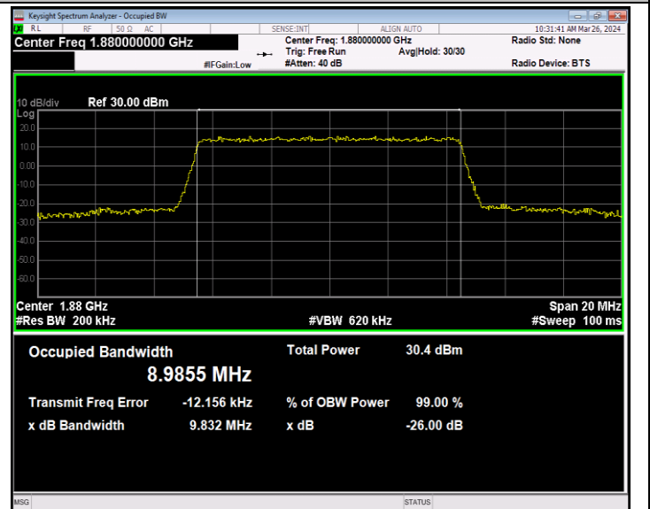
Band2-10MHz-16QAM-18900-50RB#0-PASS
