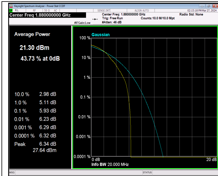
Band2-20MHz-64QAM-18900-1RB#0-PASS
