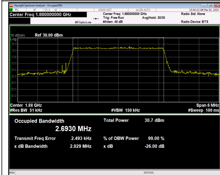
Band2-3MHz-QPSK-18900-15RB#0-PASS
