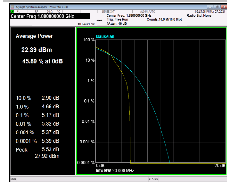
Band2-20MHz-16QAM-18900-1RB#0-PASS
