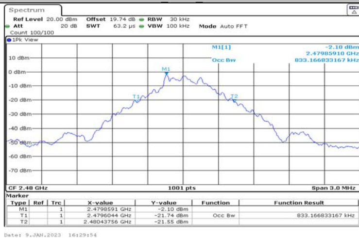
DH1_Ant1_2480
