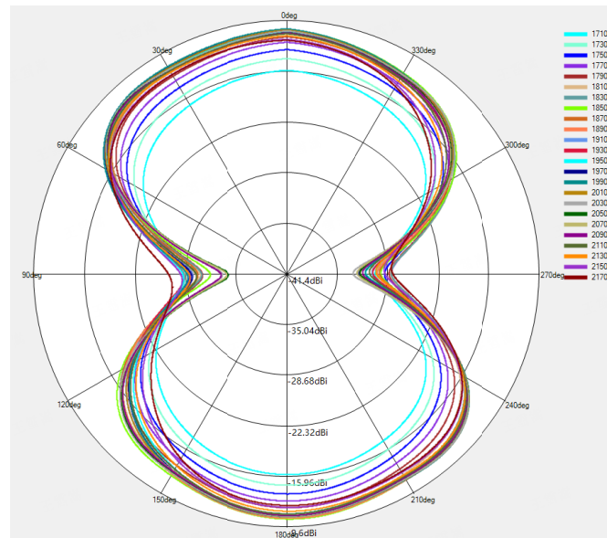
LTE B1/B2/B3 \Phi=0^\circ
