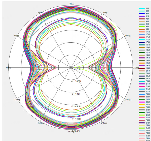
850/WCDMA B8/ LTE B8/38/41 NR n8/n38/n41 \Phi=0^\circ
