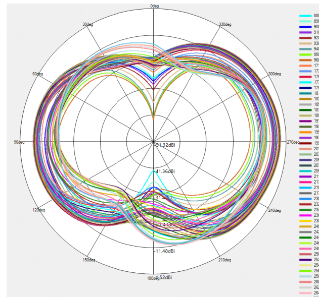
850/WCDMA B8/ LTE B8/38/41 NR n8/n38/n41 \Phi=90^\circ
