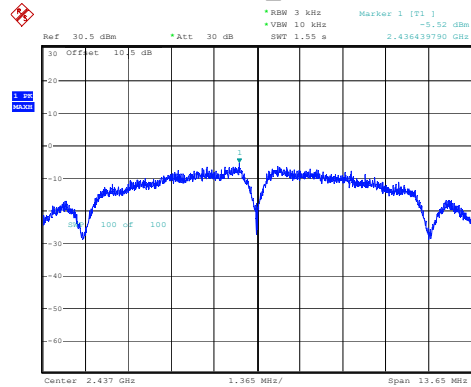
802.11b_2437MHz
