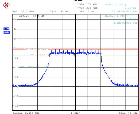
802.11g_2437MHz
