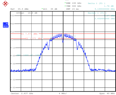
802.11b_2437MHz
