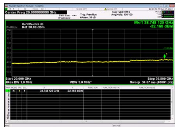
n77(60M)_DFT-s-OFDM_BPSK_ Edge_1RB_Left_634666_CH
