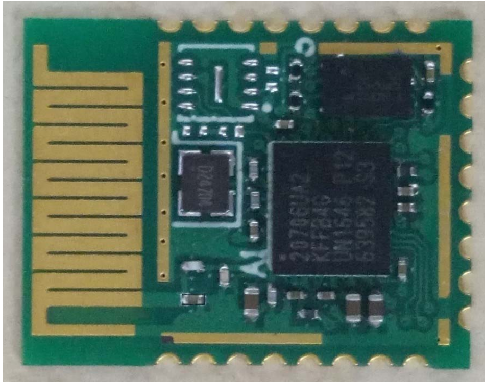
(2) EUT Photo
