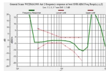
WCDMA1900 – Antenna 2
