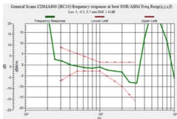
CDMA800 (BC10)
