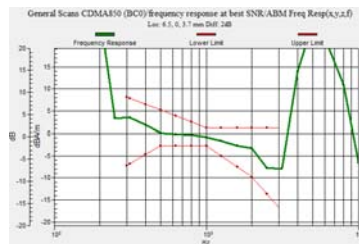
CDMA850 (BC0)
