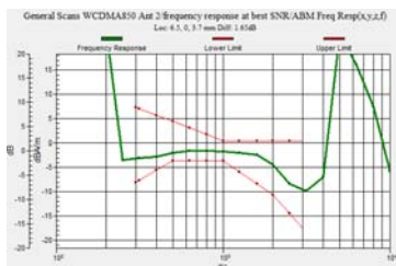
WCDMA850 – Antenna 2
