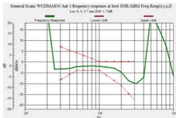
WCDMA850 – Antenna 1
