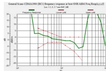
CDMA1900 (BC1)
