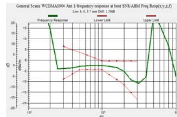
WCDMA1900 – Antenna 1
