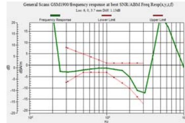
GSM1900
