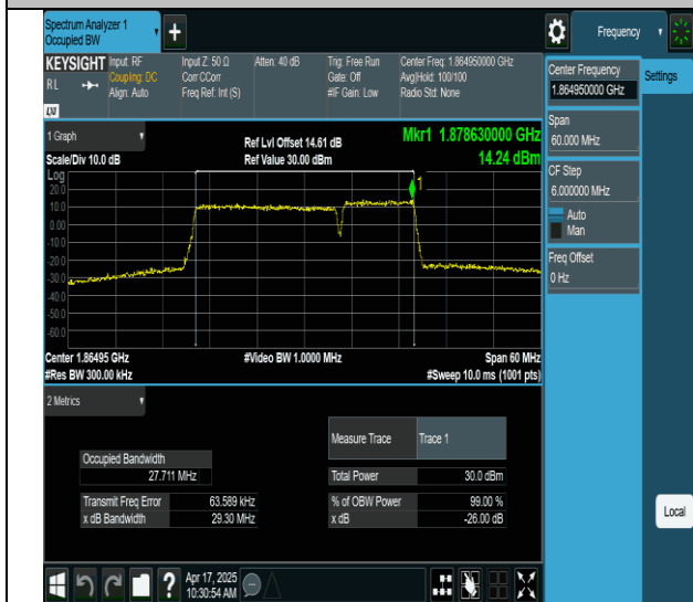
2-2-20MHz-10MHz-64QAM-64QAM-18700-18844-100RB#0-50RB#0-PASS
