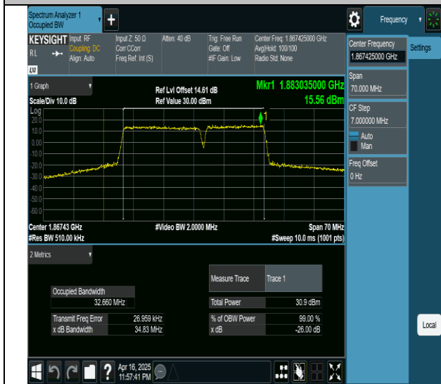
2-2-20MHz-15MHz-QPSK-QPSK-18700-18871-100RB#0- 75RB#0-PASS
