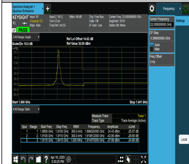
2-2-20MHz-10MHz-QPSK@QPSK-QPSK-19001-19145- 1RB#99@0RB#0-0RB#0@0RB#0-PASS
