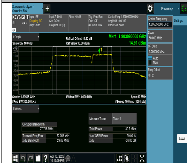
2-2-20MHz-10MHz-QPSK-QPSK-19001-19145-100RB#0-50RB#0-PASS
