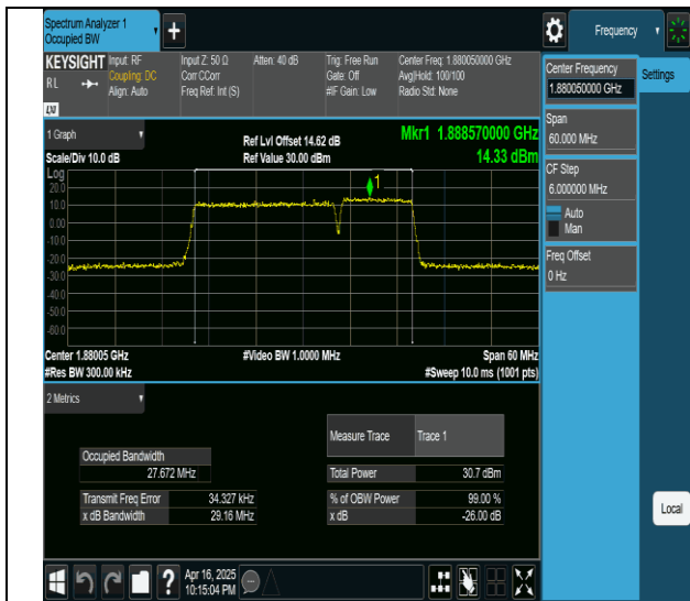
2-2-20MHz-10MHz-QPSK-QPSK-18851-18995-100RB#0-50RB#0-PASS
