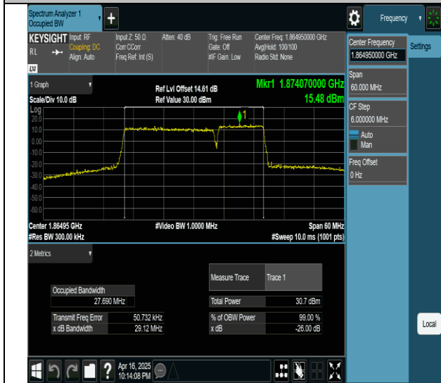
2-2-20MHz-10MHz-QPSK-QPSK-18700-18844-100RB#0-50RB#0-PASS
