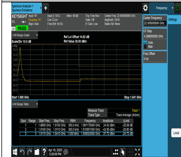
2-2-20MHz-10MHz-QPSK@QPSK-QPSK-19001-19145- 1RB#0@0RB#0-0RB#0@0RB#0-PASS
