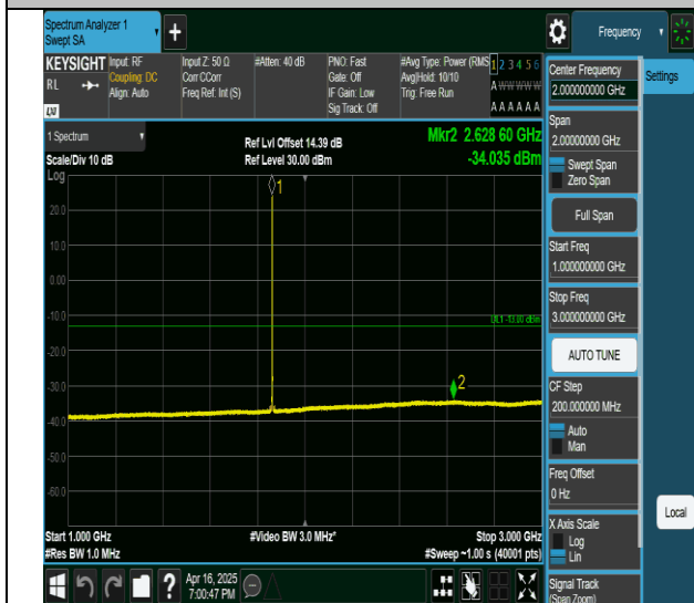
2-2-20MHz-20MHz-QPSK-QPSK-18801-18999-1RB#0-0RB#0- 1000~3000MHz-PASS
