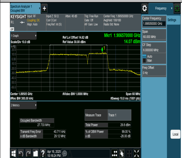
2-2-20MHz-10MHz-16QAM-16QAM-19001-19145-100RB#0-50RB#0-PASS
