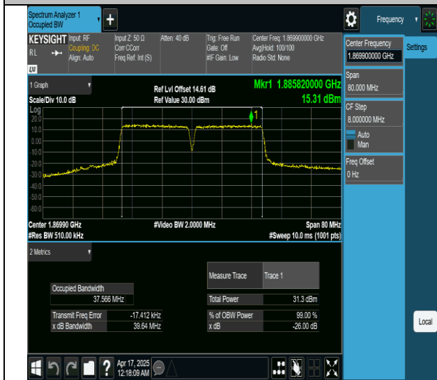
2-2-20MHz-20MHz-QPSK-QPSK-18700-18898-100RB#0-100RB#0-PASS
