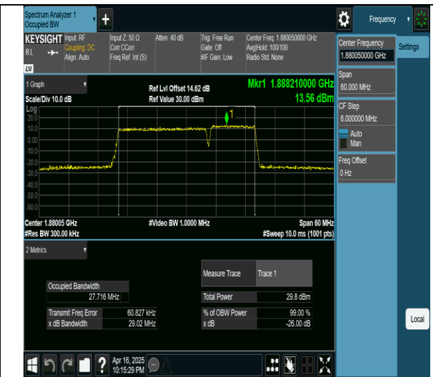
2-2-20MHz-10MHz-16QAM-16QAM-18851-18995-100RB#0-50RB#0-PASS
