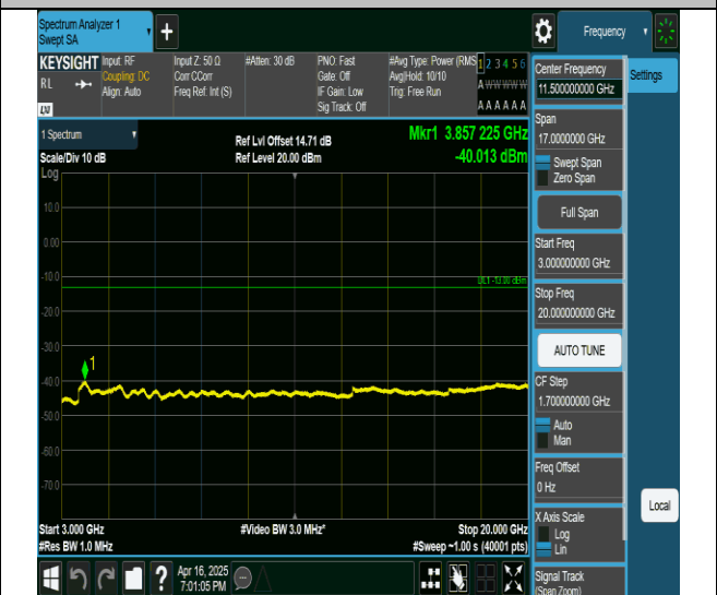
2-2-20MHz-20MHz-QPSK-QPSK-18801-18999-1RB#0-0RB#0- 3000~20000MHz-PASS
