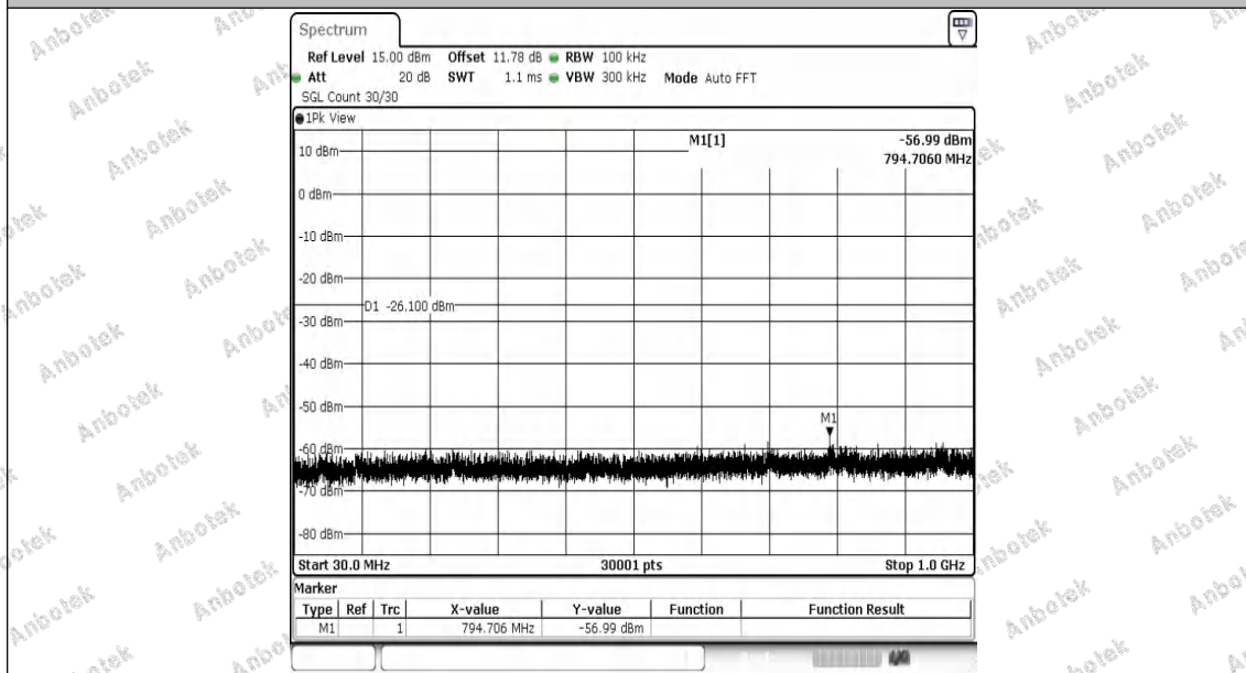
BLE_2M-Ant1-2440-30~1000-PASS
