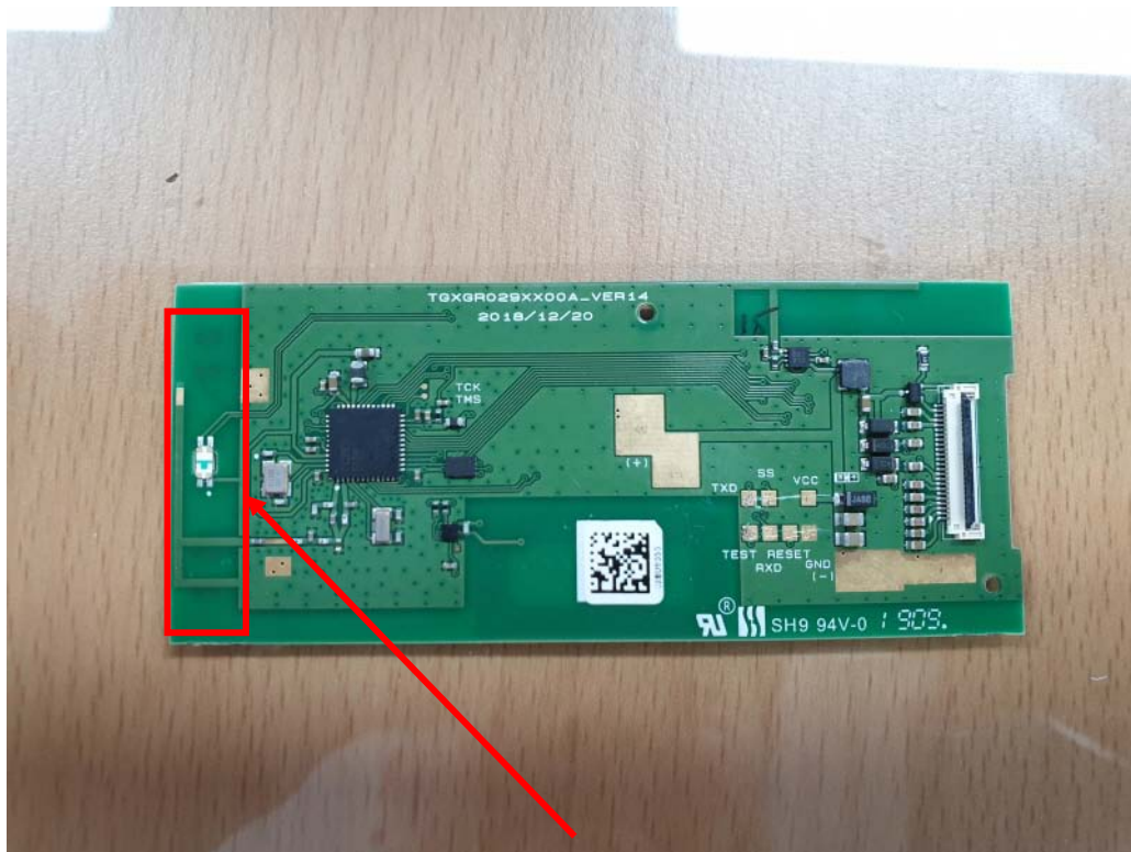
Zigbee Antenna(TX, RX)
