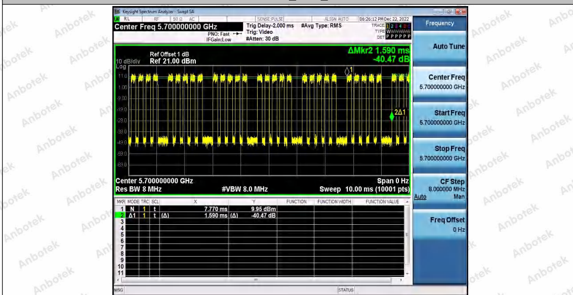
11N20SISO_Ant2_5700
