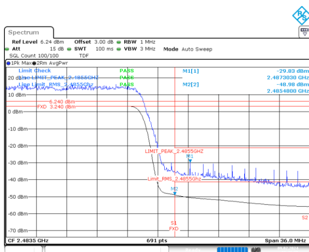
BE-R-HIGH, MIMO-A, 802.11ax20-HE0, Ch13
