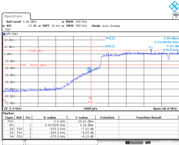
BE-NR, MIMO-A, 802.11ax40-HE0, Ch3
