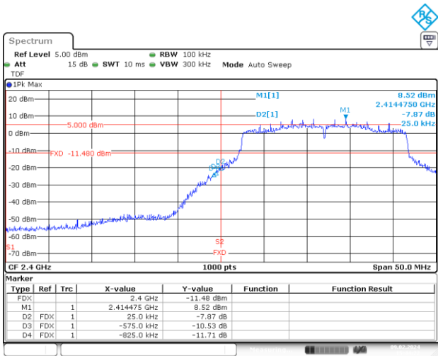
BE-NR, MIMO-A, 802.11ax20-HE0, Ch1
