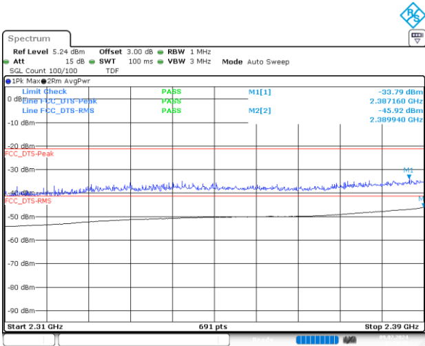
BE-R-LOW, MIMO-A, 802.11ax40-HE0, Ch3
