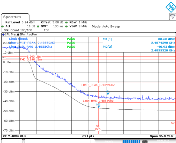
BE-R-HIGH, MIMO-A, 802.11ax40-HE0, Ch9
