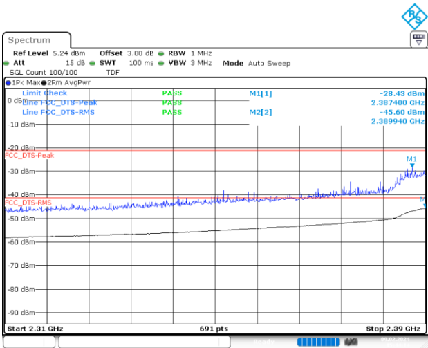
BE-R-LOW, MIMO-A, 802.11ax20-HE0, Ch1
