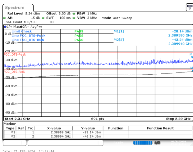
BE-R-LOW, SISO-B, 802.11ax40-HE0, Ch3
