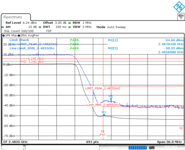
BE-R-HIGH, MIMO-A, 802.11n40-HT8, Ch11
