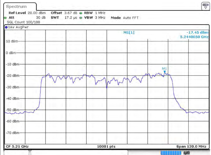
PSDac80 5210MHz Ant1
