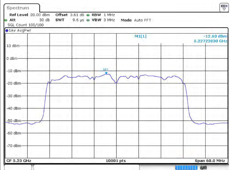
PSDac40 5230MHz Ant1
