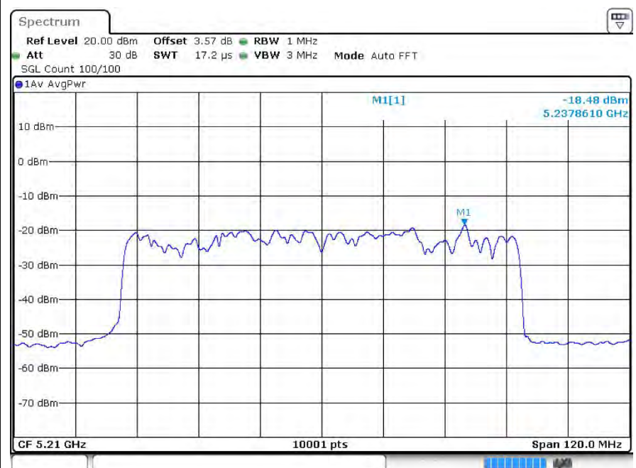
PSDac80 5210MHz Ant2
