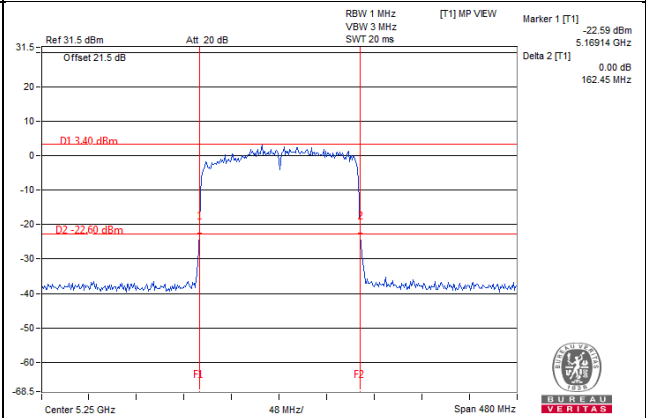
802.11ax (HE160)_Chain 2 / CH50 (U-NII-2A)
