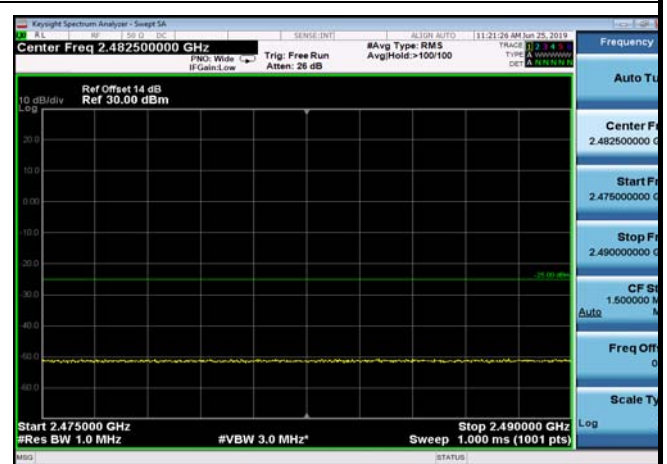
FDD07_5MHz_2567.5_QPSK_OneRB_low _ExtraBands_Range_2475~2490
