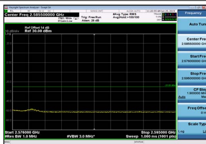
FDD07_5MHz_2567.5_Q16_OneRB_high _ExtraBands_Range_2576~2595
