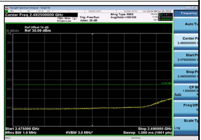
FDD07_15MHz_2507.5_Q16_fullRB_ExtraBands_Range_2475~2490
