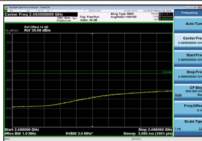
FDD07_10MHz_2505_Q16_fullRB_ExtraBand s_Range_2490~2496
