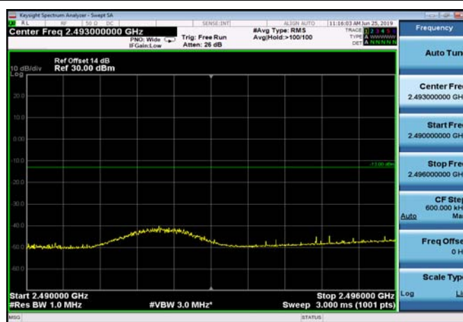
FDD07_20MHz_2510_Q16_OneRB_low _ExtraBands_Range_2490~2496
