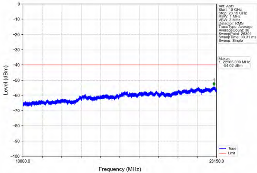
Band30_10MHz_QPSK_MCH_2310MHz_RB_1_49_NTNV
