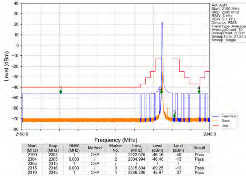
Band30_10MHz_QPSK_MCH_2310MHz_RB_1_0_NTNV
