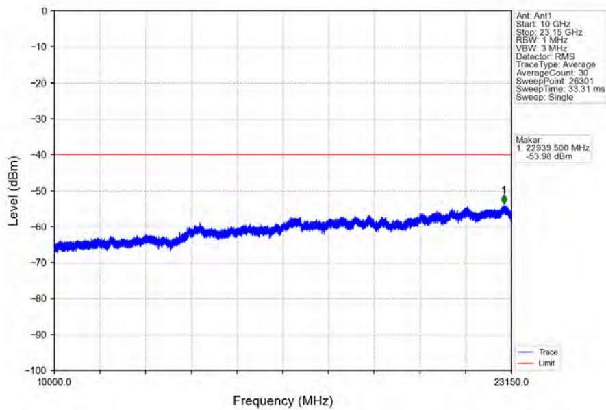
Band30_10MHz_QPSK_LCH_2310MHz_RB_50_0_NTNV
