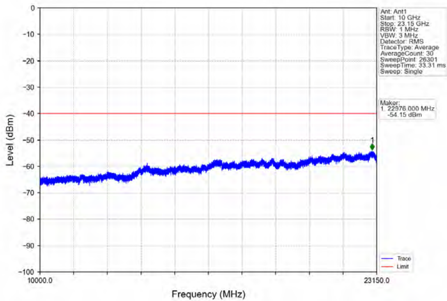
Band30_5MHz_QPSK_LCH_2307.5MHz_RB_25_0_NTNV
