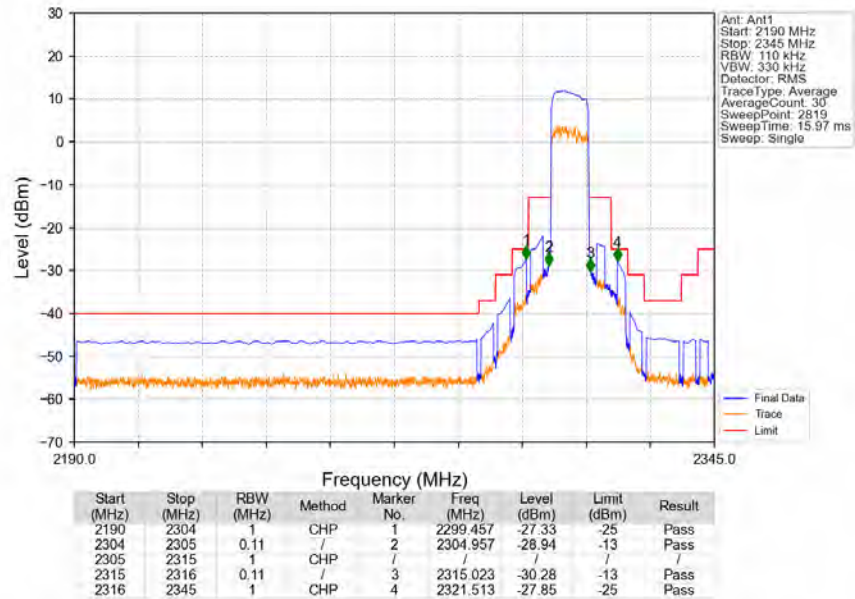
Band30_10MHz_QPSK_HCH_2310MHz_RB_1_0_NTNV
