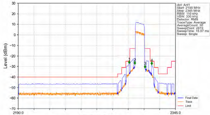
Band30_10MHz_QPSK_HCH_2310MHz_RB_50_0_NTNV
