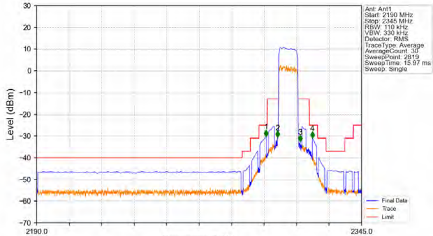
Band30_10MHz_16QAM_LCH_2310MHz_RB_50_0_NTNV
