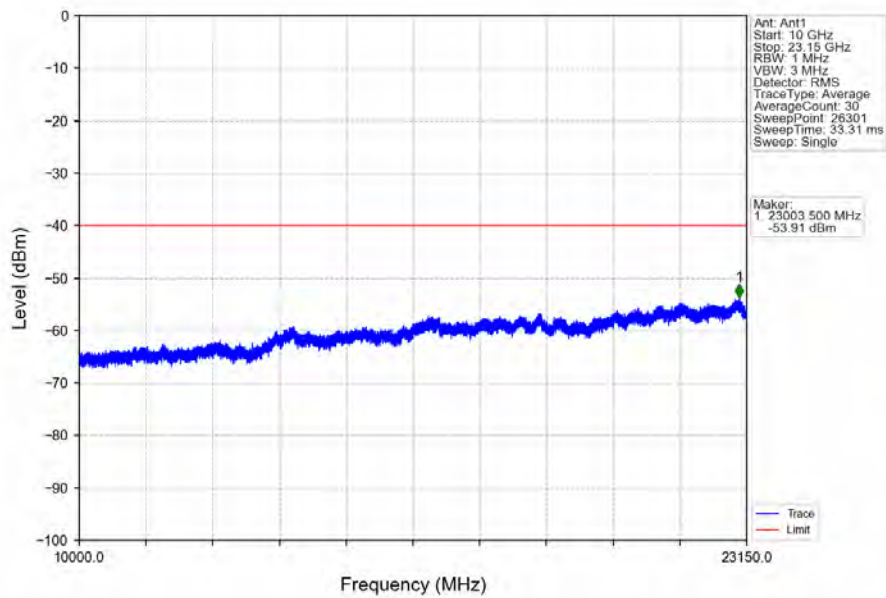
Band30_10MHz_QPSK_HCH_2310MHz_RB_1_49_NTNV
