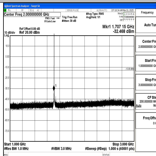
Band4 1.4MHz QPSK 19957 1RB#0 1000~3000 1000~3000
