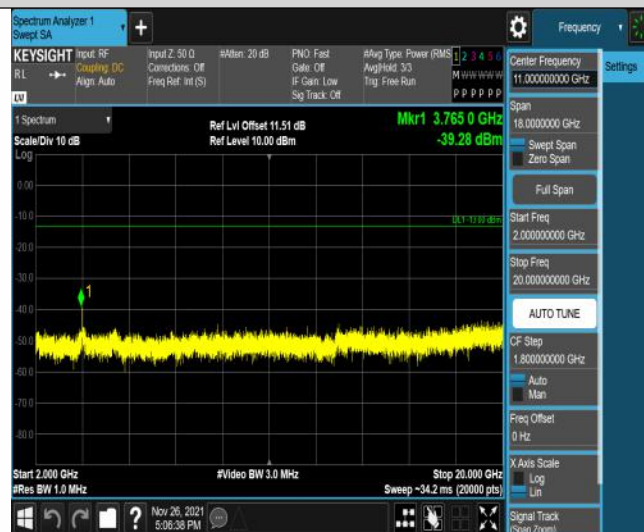
Band25-10MHz-QPSK-26365-50RB#0-Range3:2000~20000MHz
