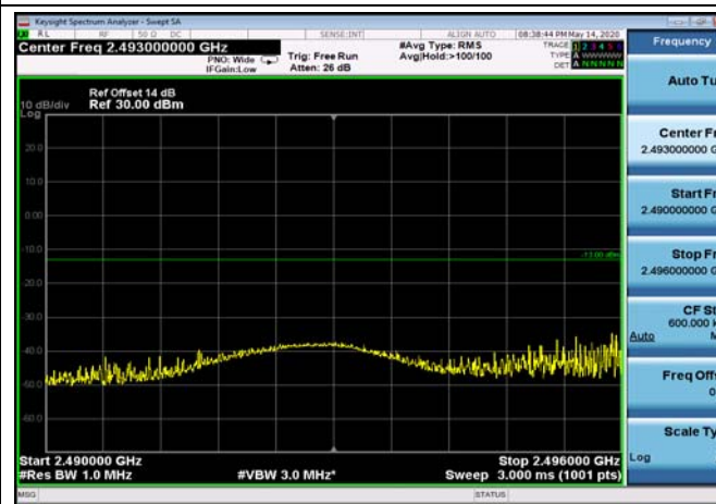
FDD07_20MHz_2510_Q16_OneRB_low _ExtraBands_Range_2490~2496
