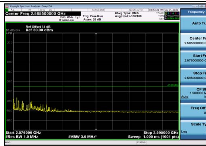
FDD07_5MHz_2567.5_Q16_OneRB_high _ExtraBands_Range_2576~2595
