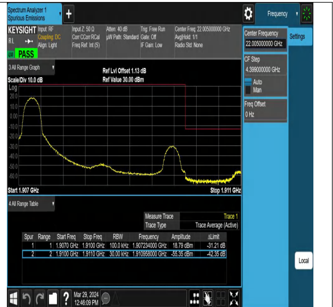
Band2_3MHz_QPSK_19185_1RB#0
