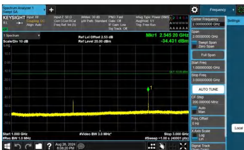
Band26(824-849)-10MHz-QPSK-26990-1RB#49-1000~3000-PAS
