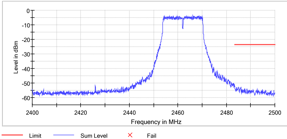
Band Edge
