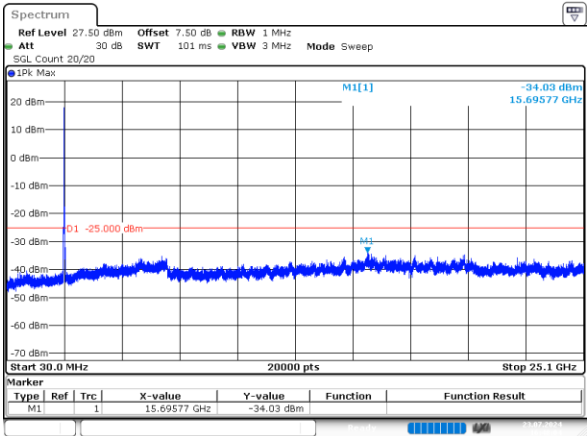
20MHz_Low_QPSK_100@0 -34.03dBm
