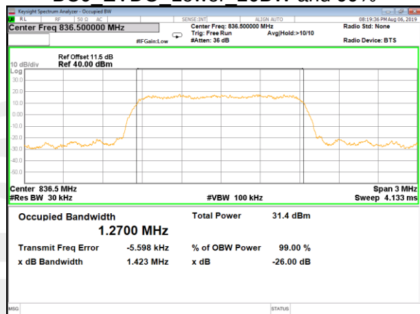
BC0_EVDO_Middle_26BW and 99%
