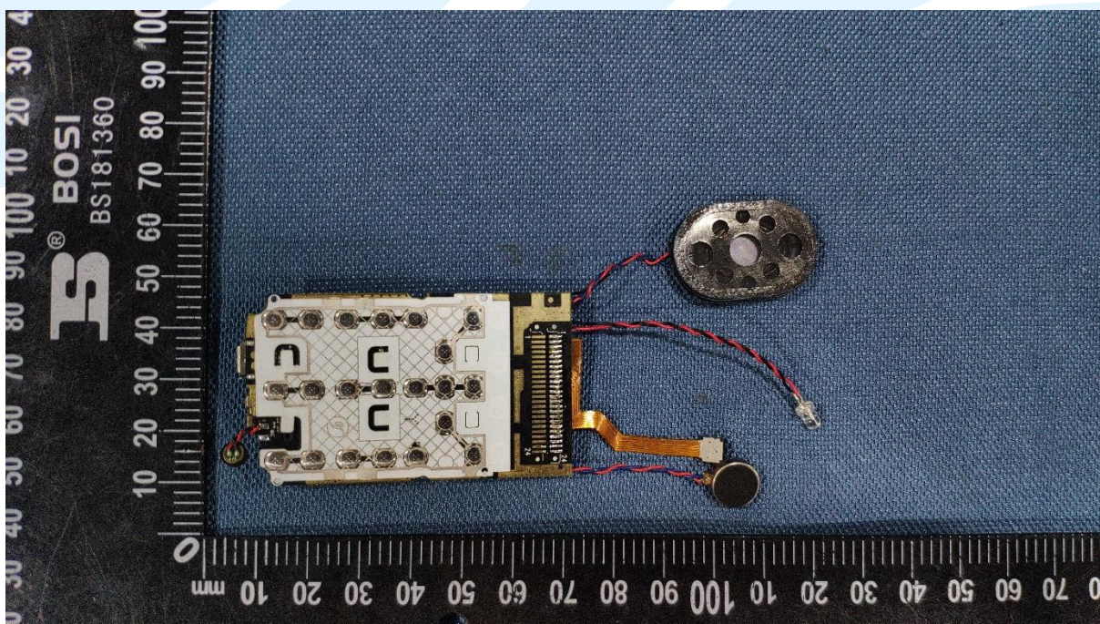
EUT Photo
