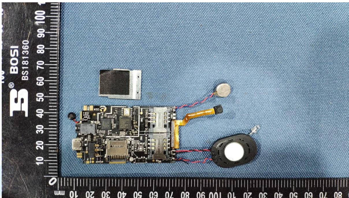
EUT Photo
