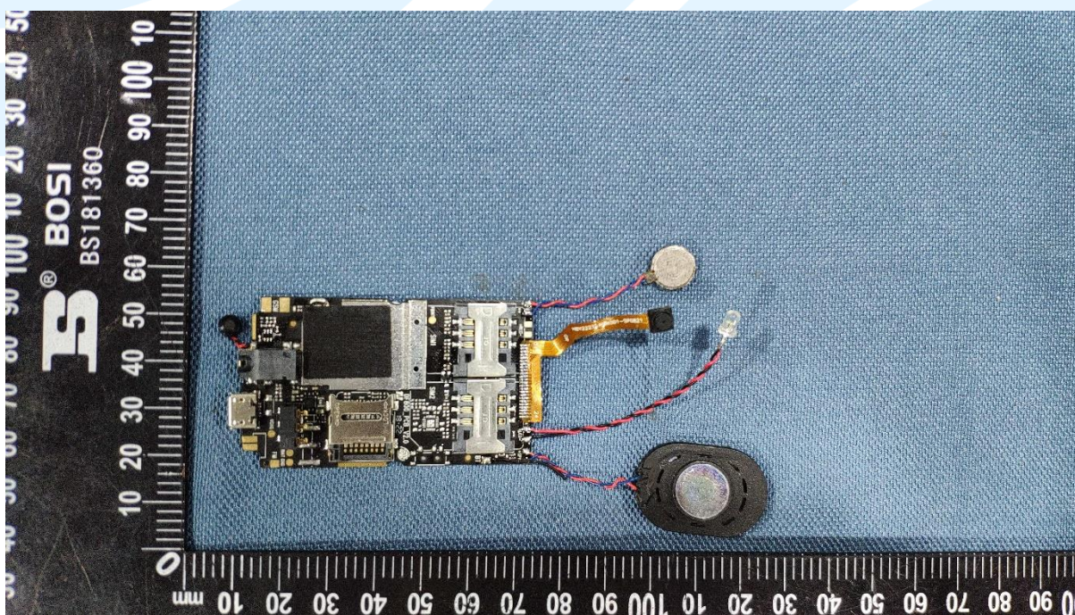
EUT Photo
