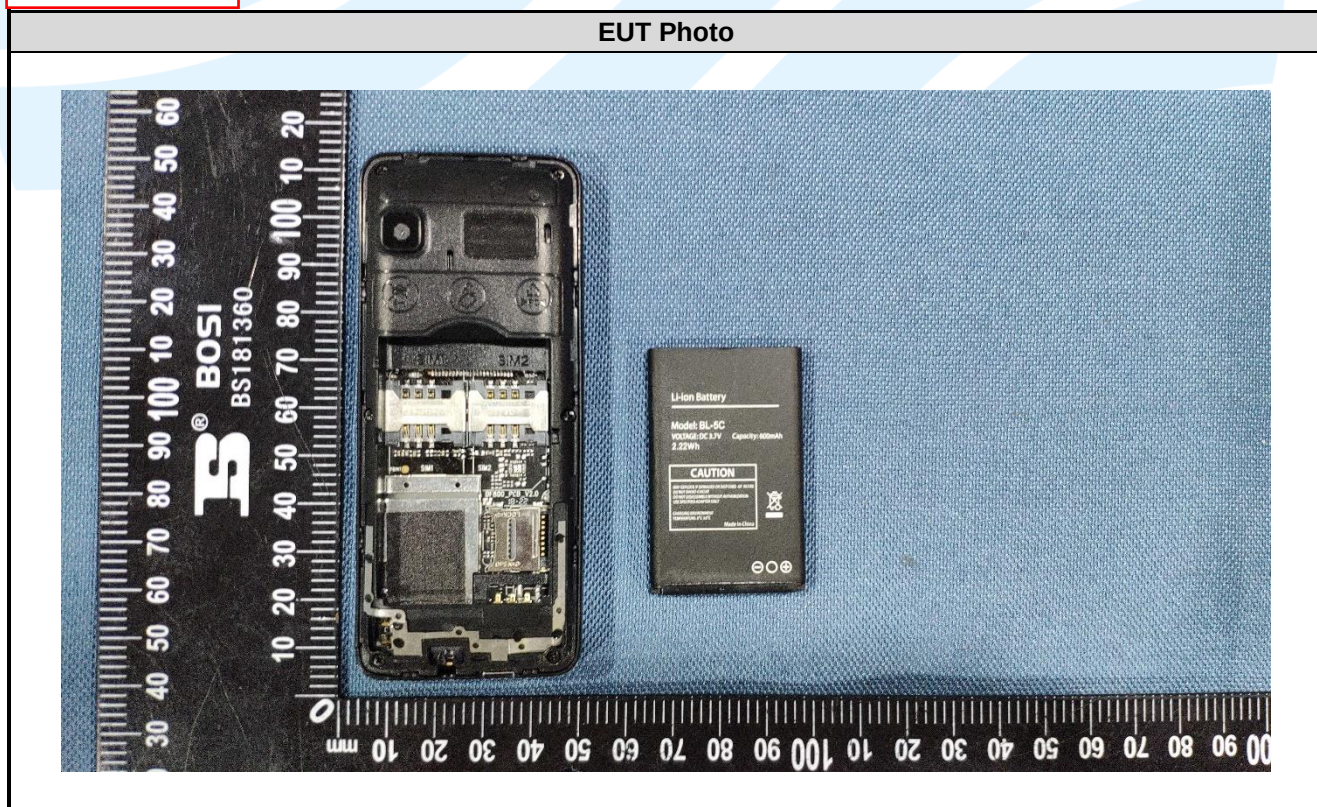
GSM Antenna
