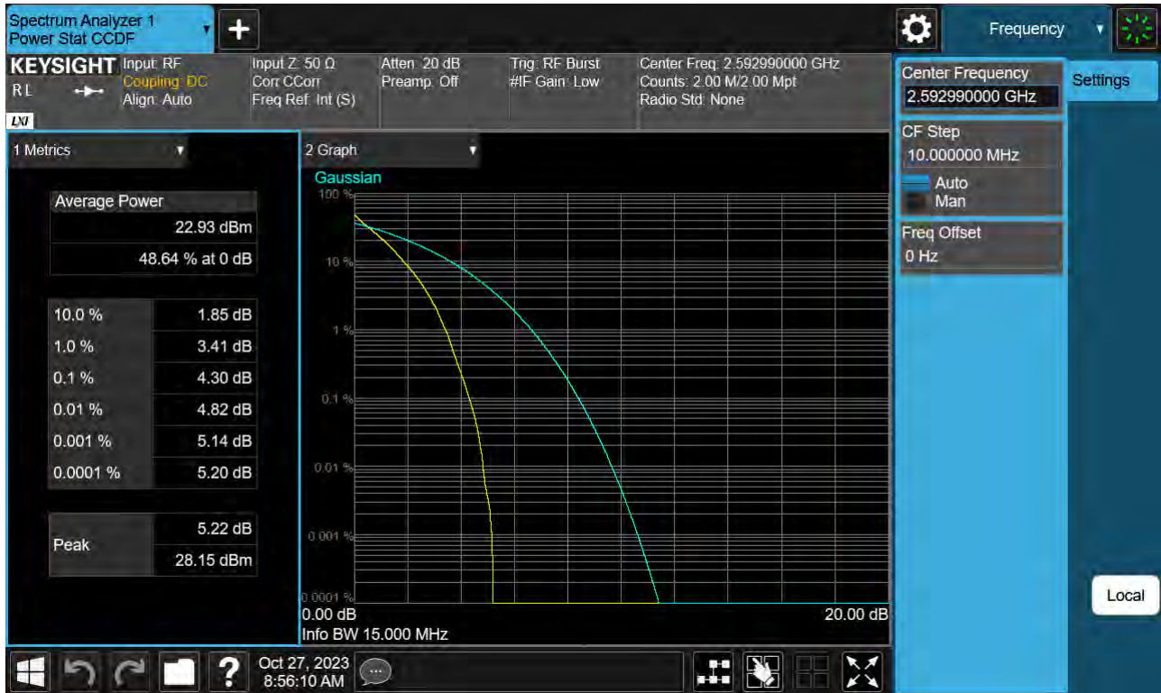
Sub6 n41. PAR Plot (15 M BW_Ch.518598_BPSK)
