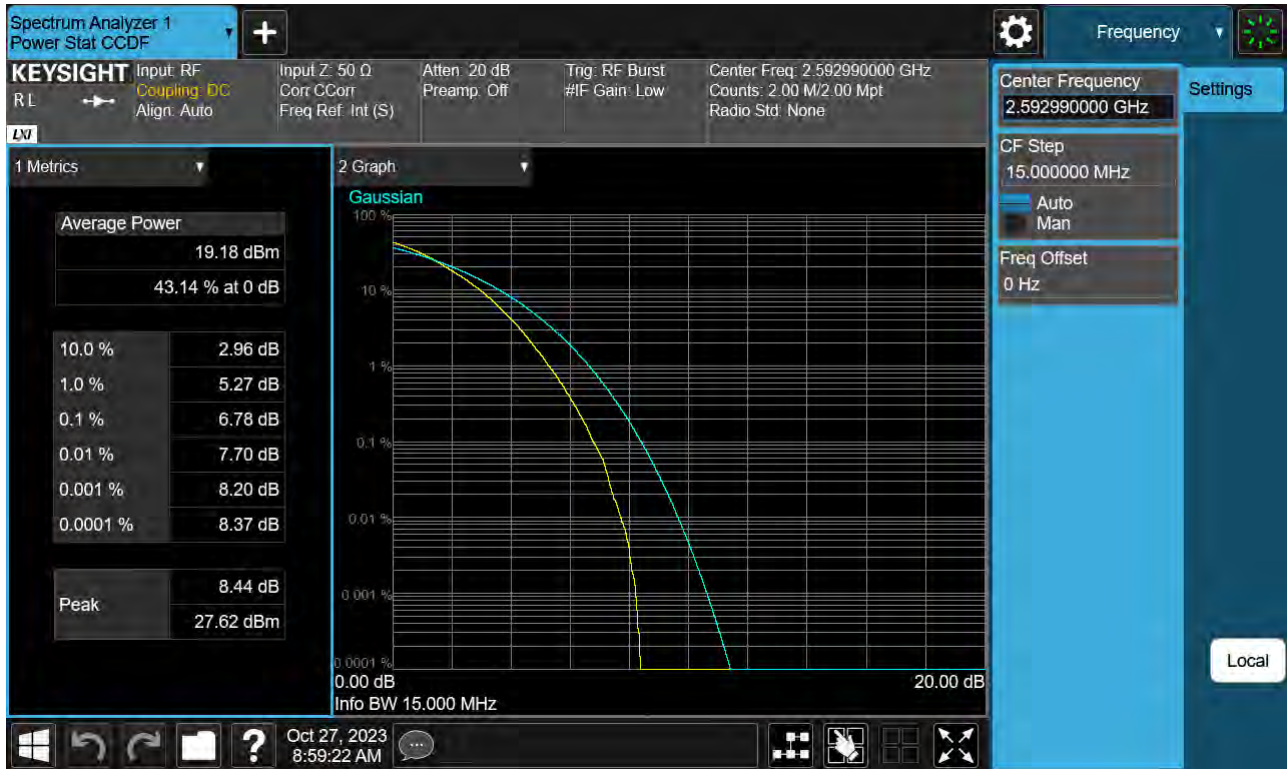
Sub6 n41. PAR Plot (15 M BW_Ch.518598_256QAM)
