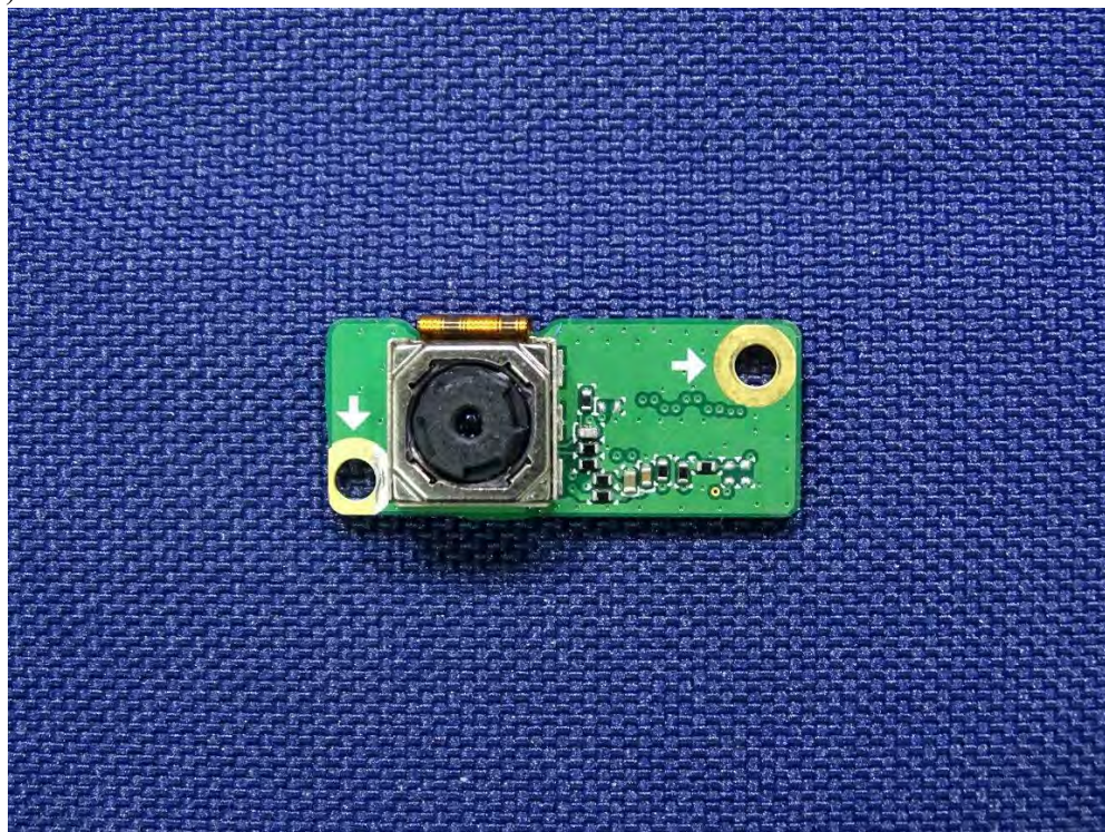
(36) EUT Photo
