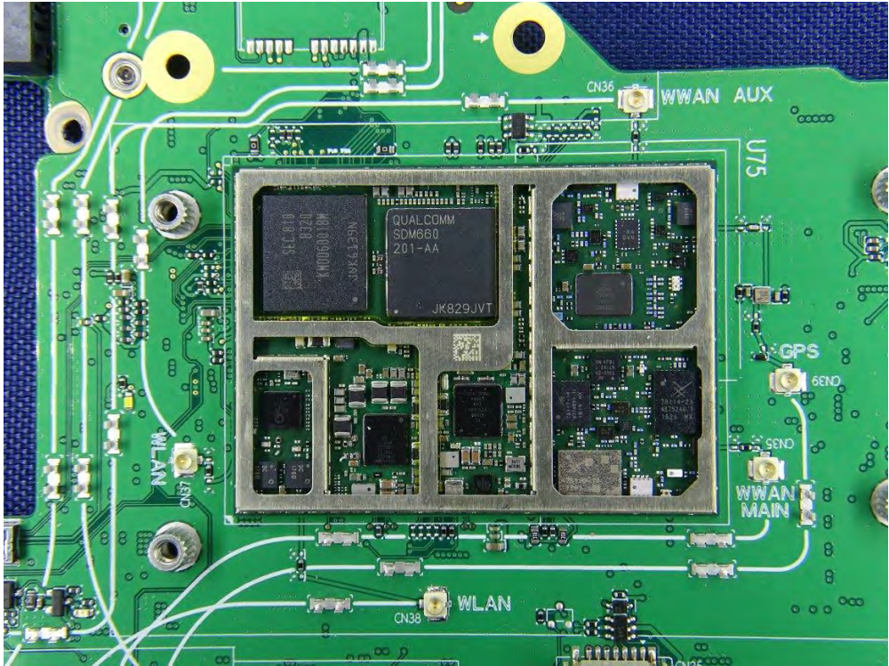
(39) EUT Photo - Module
