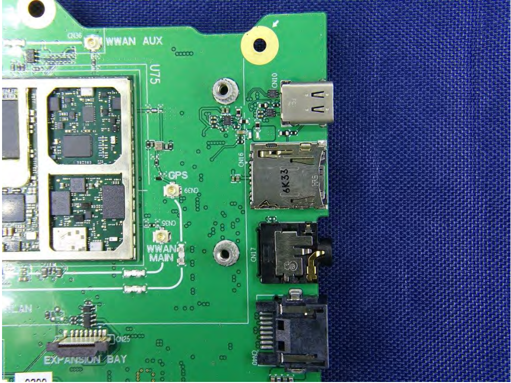
(40) EUT Photo
