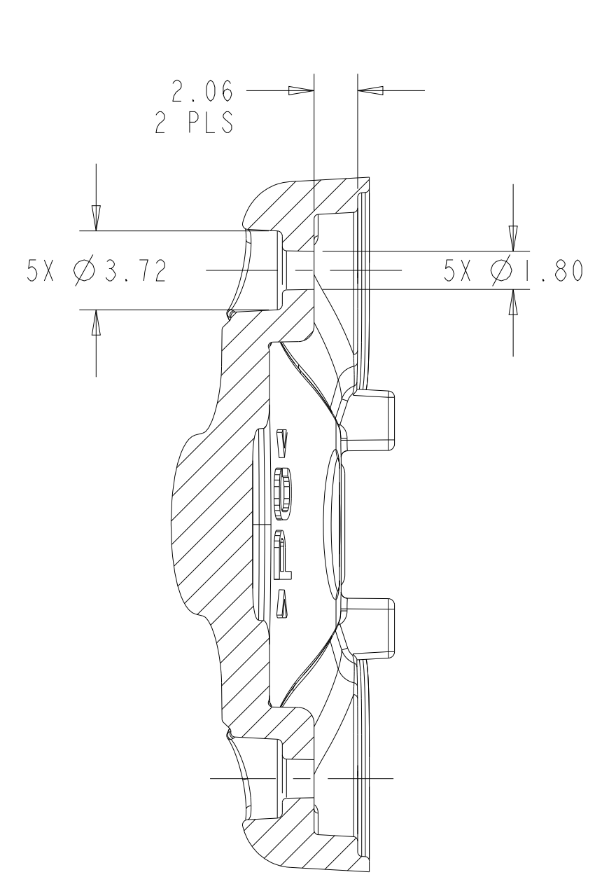
SECTION D-D
