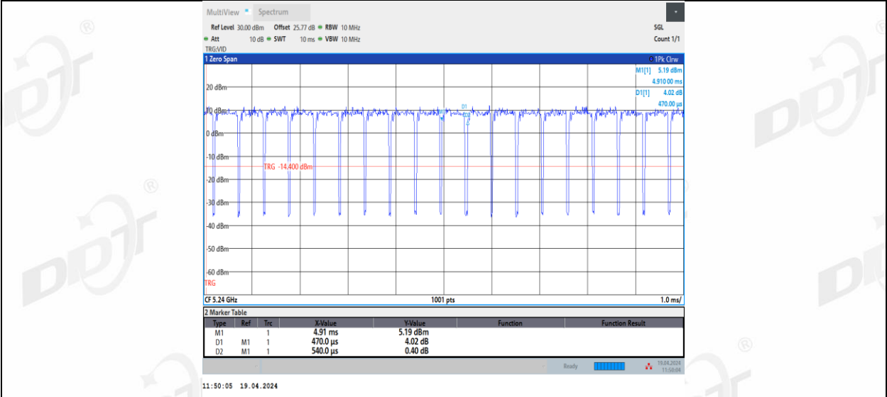
11N20MIMO_Ant3_5240
