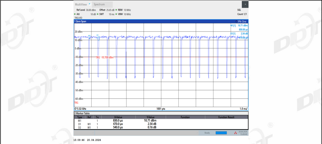
11N20MIMO_Ant3_5320
