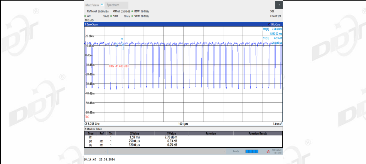
11N40MIMO_Ant3_5755
