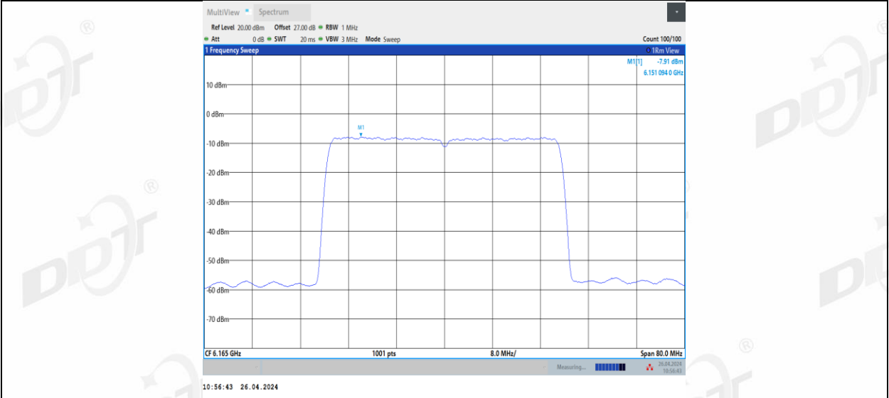
11AX40MIMO_Ant3_6165
