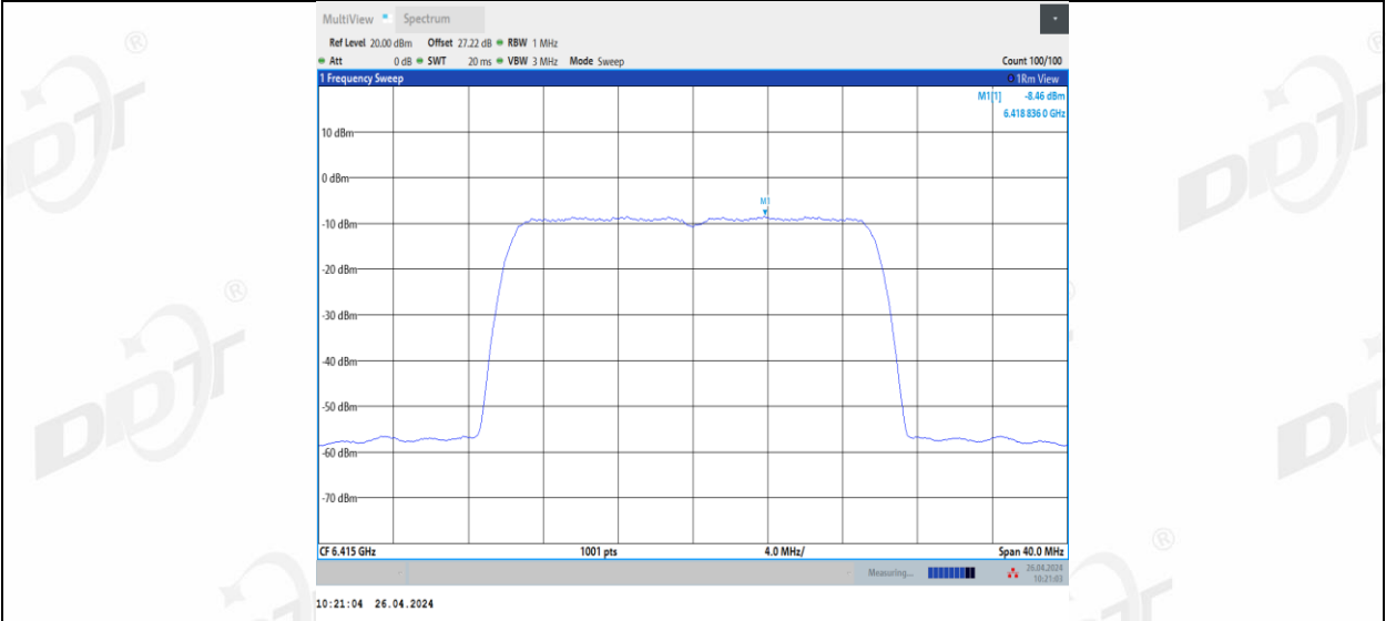
11AX20MIMO_Ant3_6415
