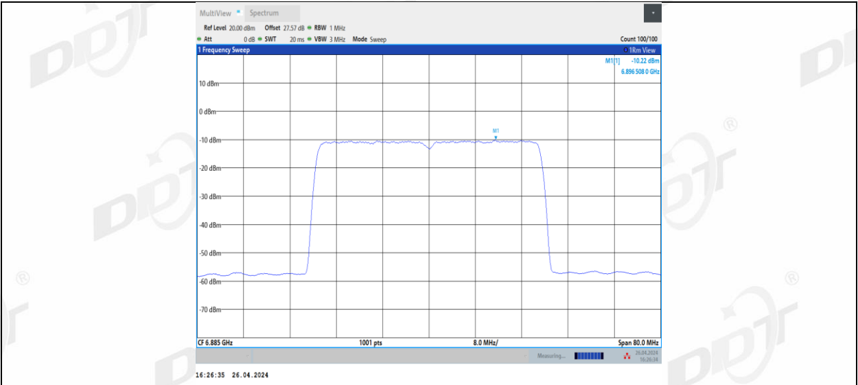
11AX40MIMO_Ant2_6885
