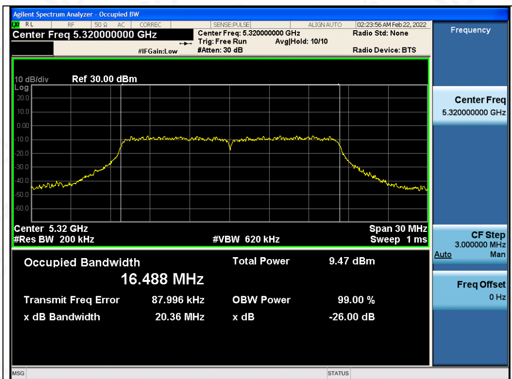
Test_Graph_802.11a_ANT1_5320_6Mbps_OBW
