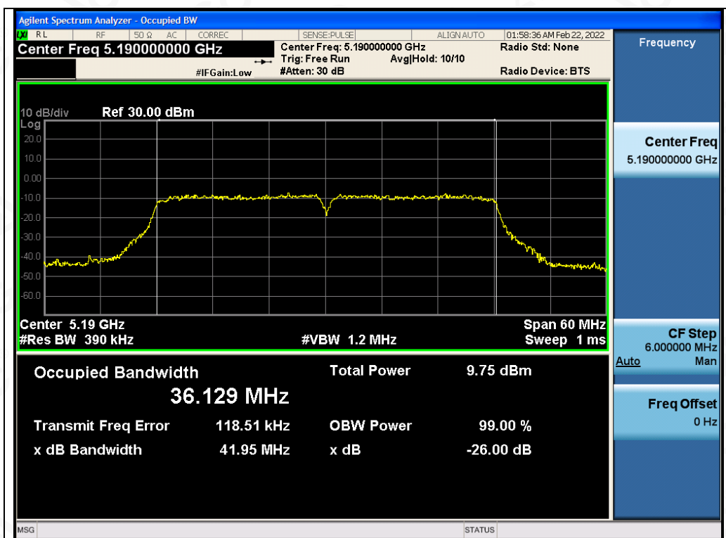
Test_Graph_802.11n40_ANT1_5190_MCS0_OBW
