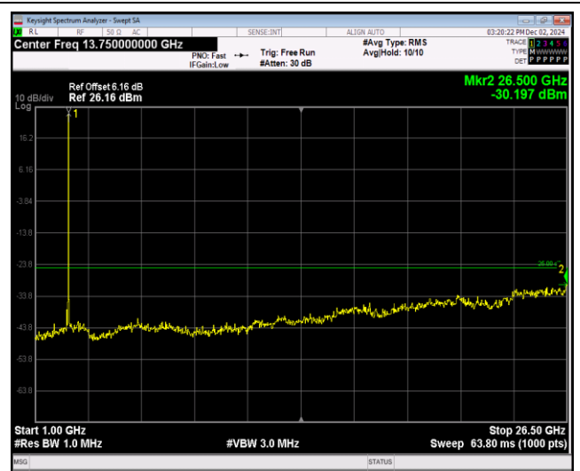
Band38-20MHz-64QAM-37850-1RB#0-Range2:1000~26500MHz
