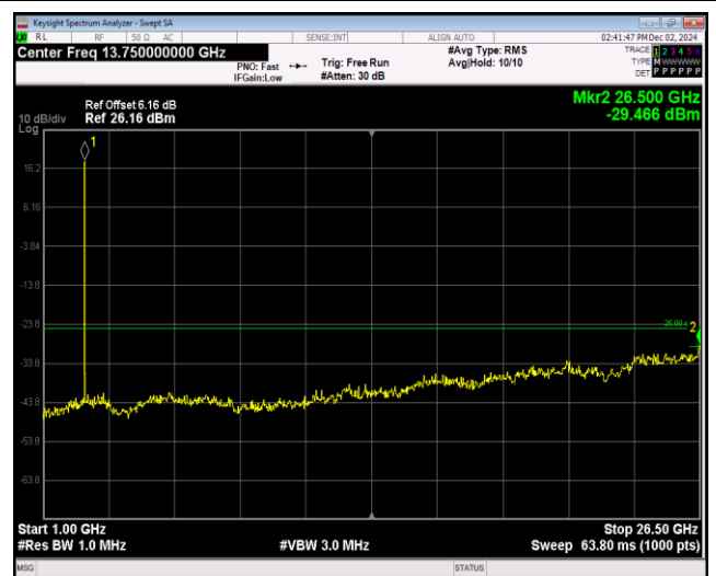
Band38-20MHz-QPSK-37850-1RB#0-Range2:1000~26500MHz
