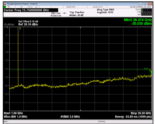
Band38-5MHz-QPSK-38000-1RB#0-Range2:1000~2 6500MHz
