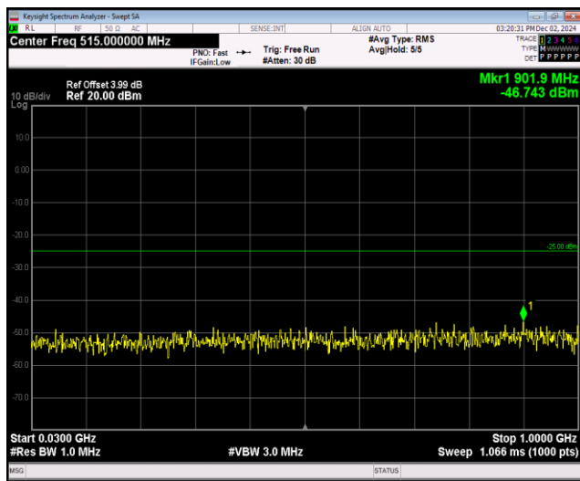
Band41-5MHz-QPSK-40065-1RB#0-Range1:30~1000MHz
