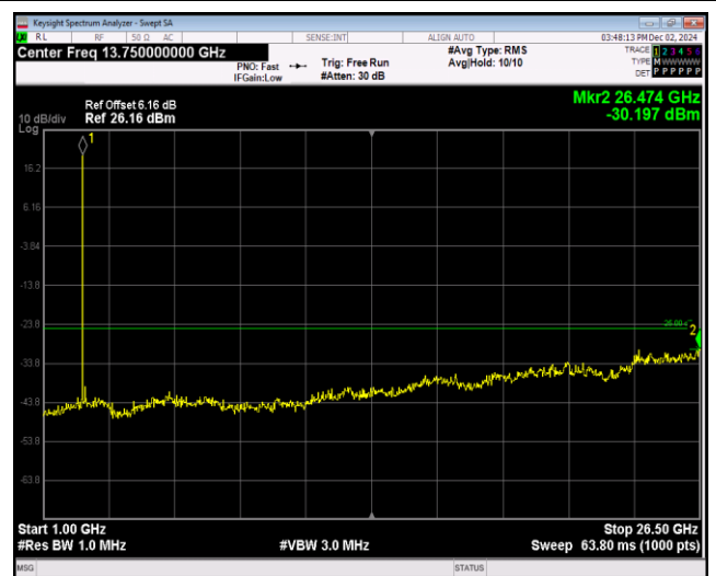
Band41-5MHz-QPSK-40640-1RB#0-Range2:1000~26500MHz
