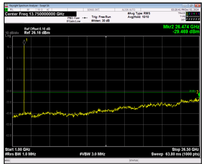
Band41-5MHz-QPSK-40065-1RB#0-Range2:1000~26500MHz
