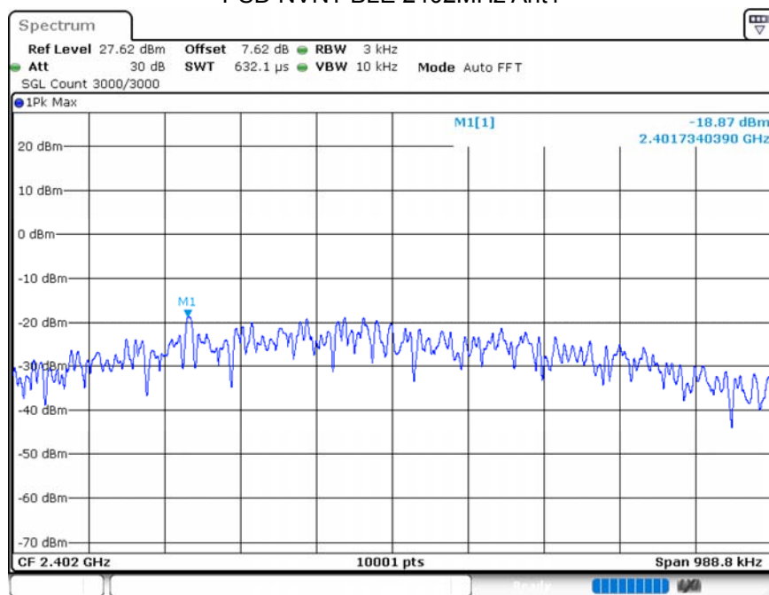
PSD NVNT BLE 2402MHz Ant1
