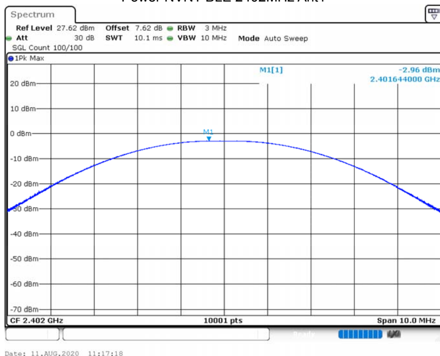
Power NVNT BLE 2402MHz Ant1
