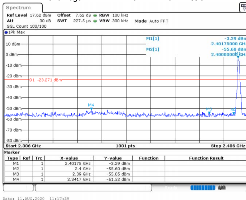
Band Edge NVNT BLE 2402MHz Ant1 Emission
