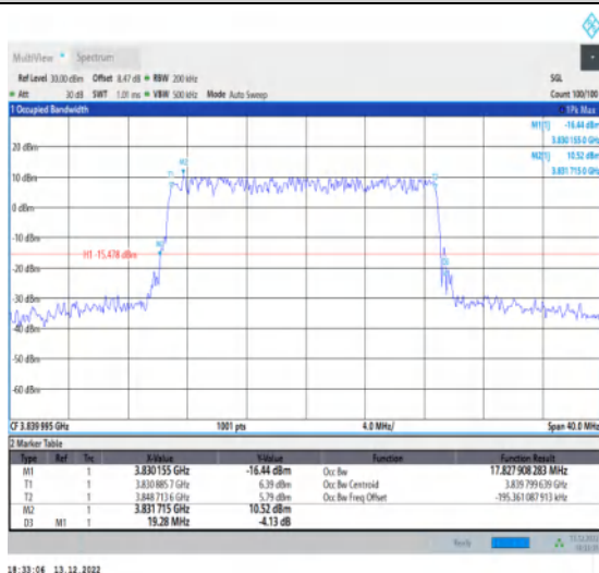
1-N77-3700-3980-30-20-M-4-DFT-64QAM-Outer_Ful l-50@0-Ant1-17.828-19.280-≤20-PASS
