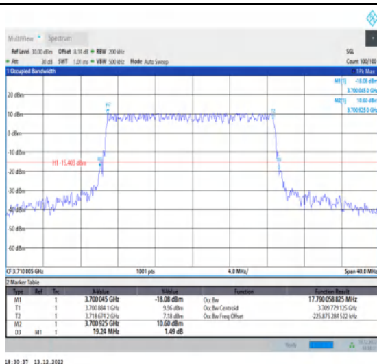
1-N77-3700-3980-30-20-L-3-DFT-16QAM-Outer_Full -50@0-Ant1-17.79-19.240-≤20-PASS
