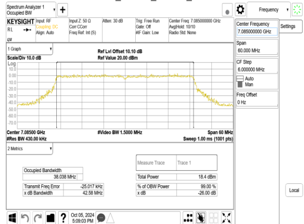
802.11be_40MHz_Chain1_7085MHz
