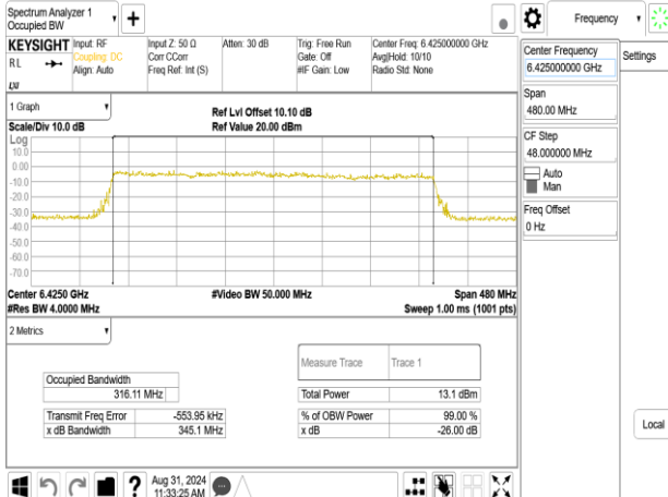
802.11be_320MHz_Chain1_6425MHz
