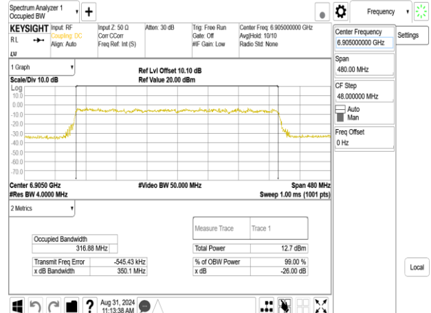
802.11be_320MHz_Chain1_6905MHz
