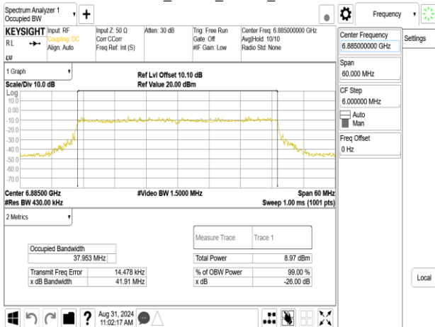
802.11be_40MHz_Chain1_6885MHz
