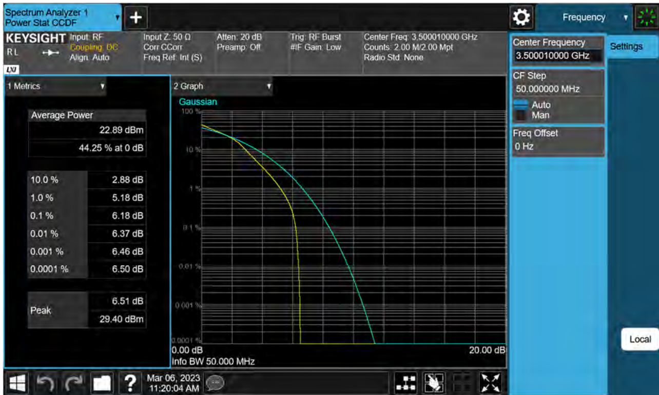
Sub6 n77(78). PAR Plot (50 M BW_Ch.633334_16QAM)
