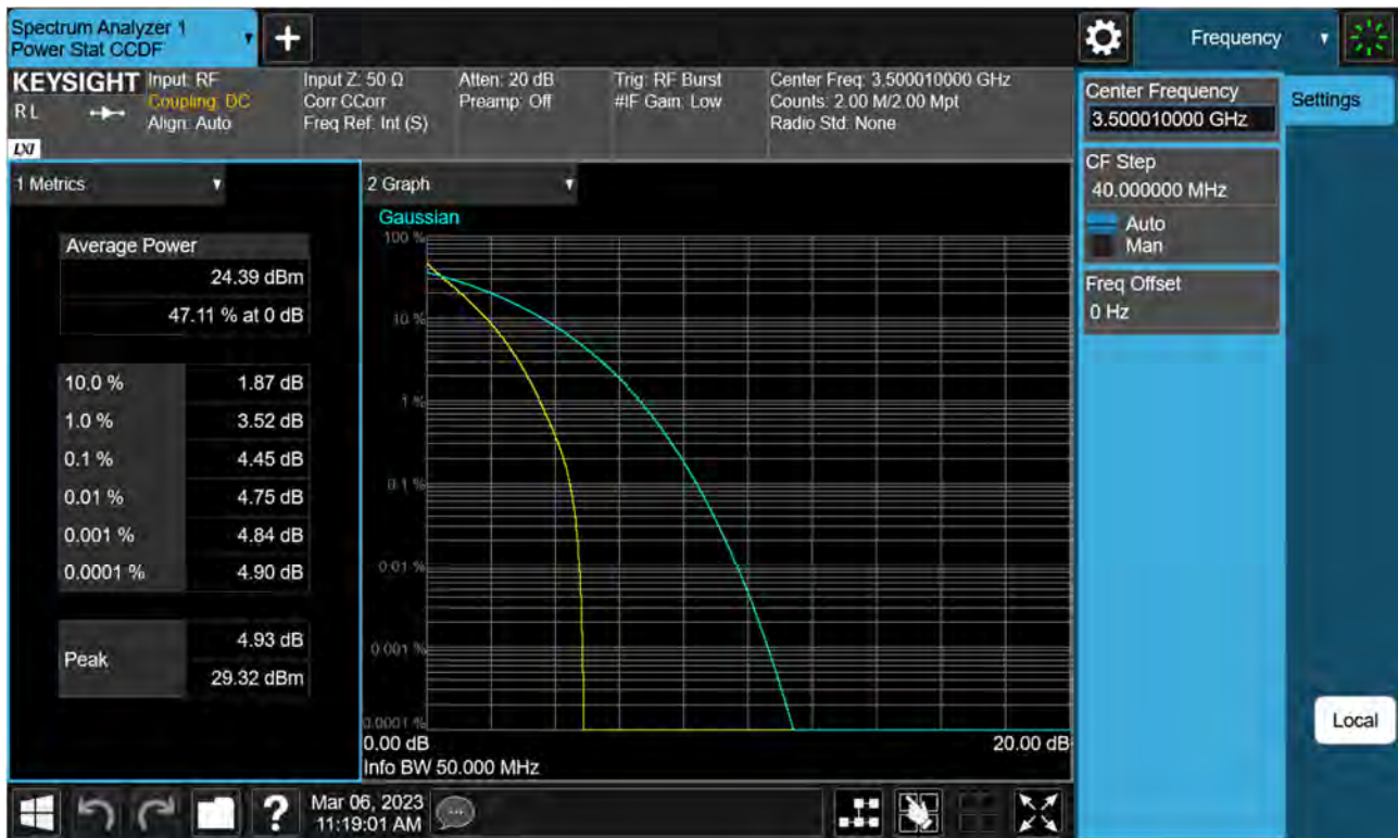
Sub6 n77(78). PAR Plot (50 M BW_Ch.633334_BPSK)
