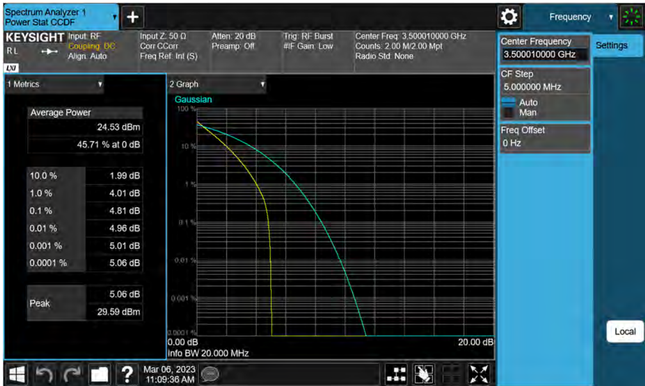
Sub6 n77(78). PAR Plot (20 M BW_Ch.633334_BPSK)
