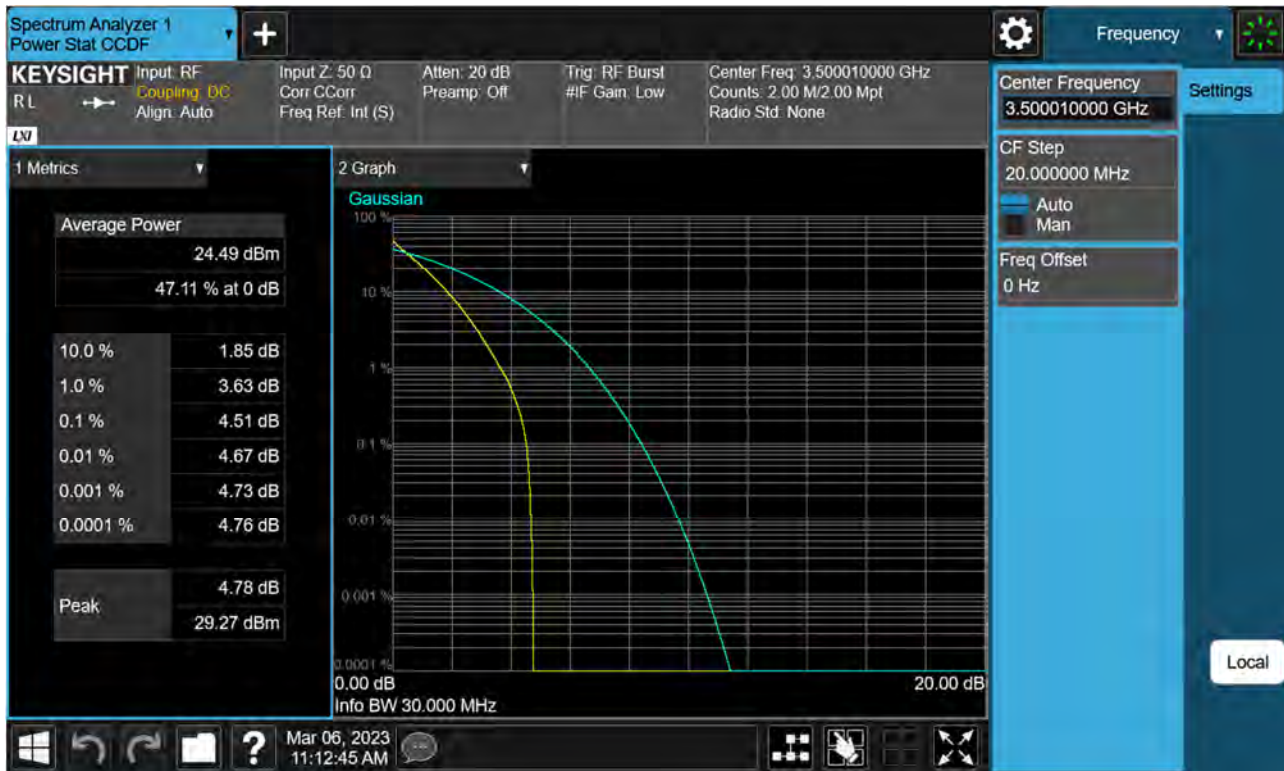
Sub6 n77(78). PAR Plot (30 M BW_Ch.633334_ BPSK)
