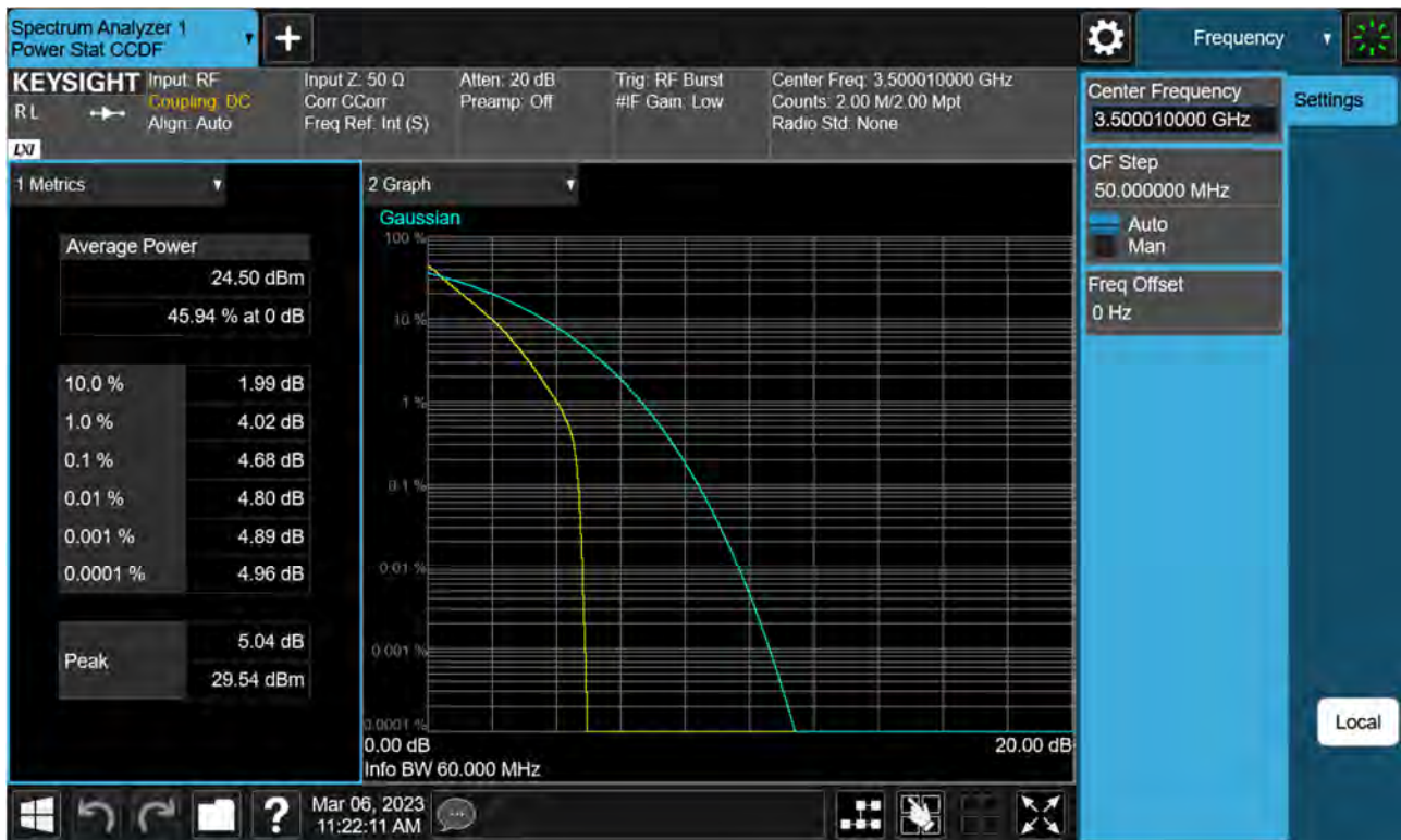
Sub6 n77(78). PAR Plot (60 M BW_Ch.633334_BPSK)
