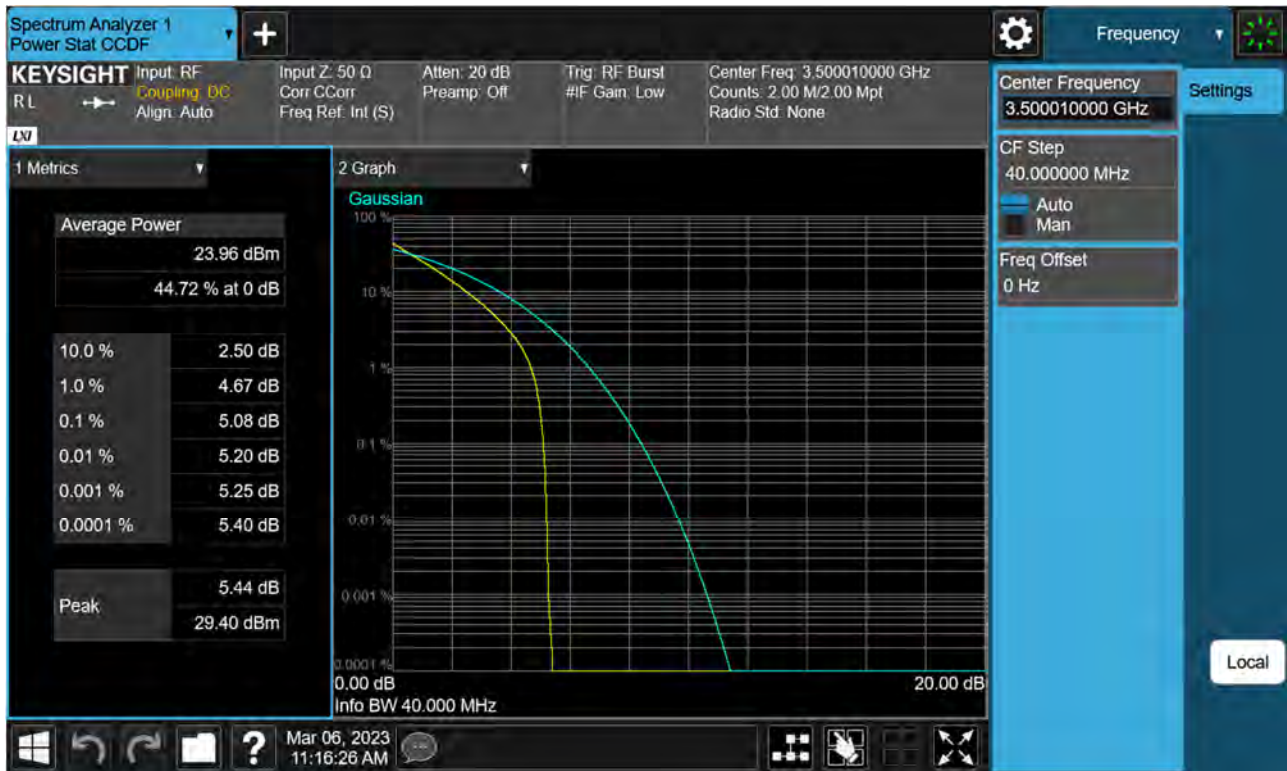
Sub6 n77(78). PAR Plot (40 M BW_Ch.633334_QPSK)
