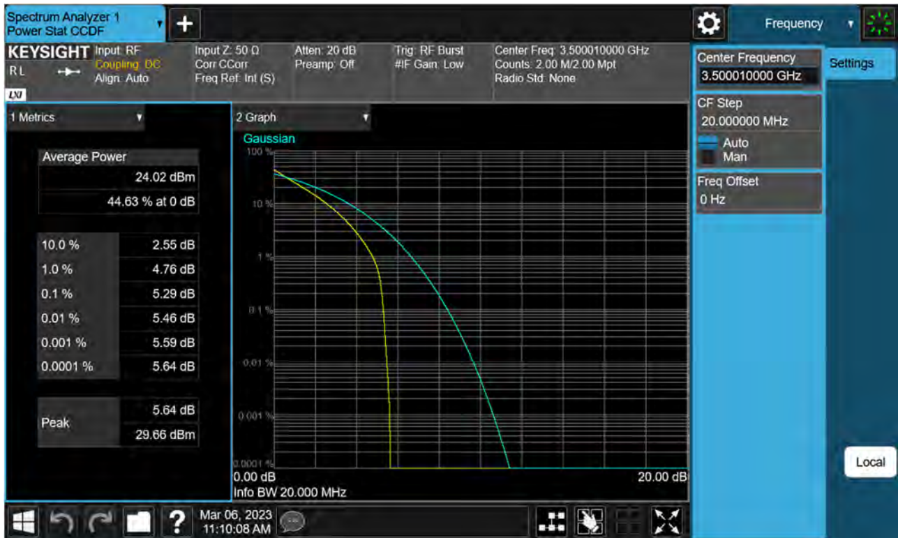
Sub6 n77(78). PAR Plot (20 M BW_Ch.633334_QPSK)
