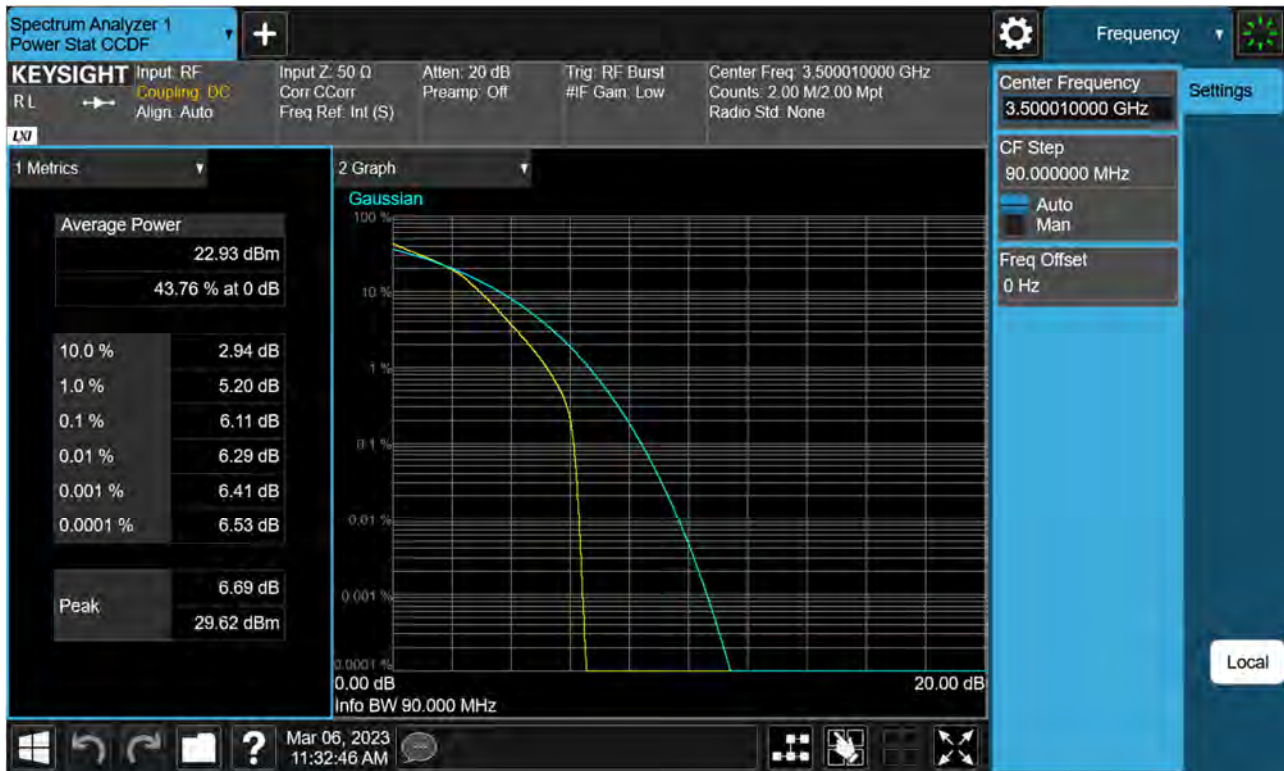
Sub6 n77(78). PAR Plot (90 M BW_Ch.633334_16QAM)
