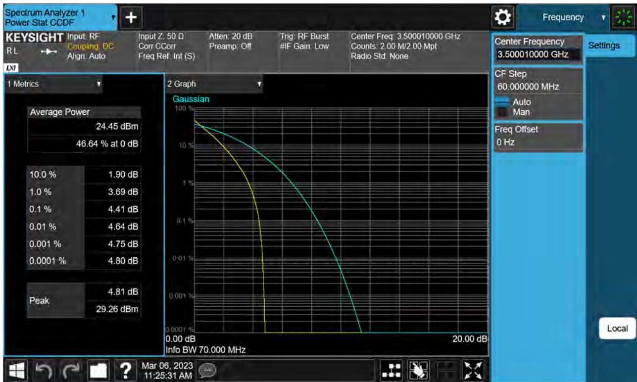
Sub6 n77(78). PAR Plot (70 M BW_Ch.633334_BPSK)
