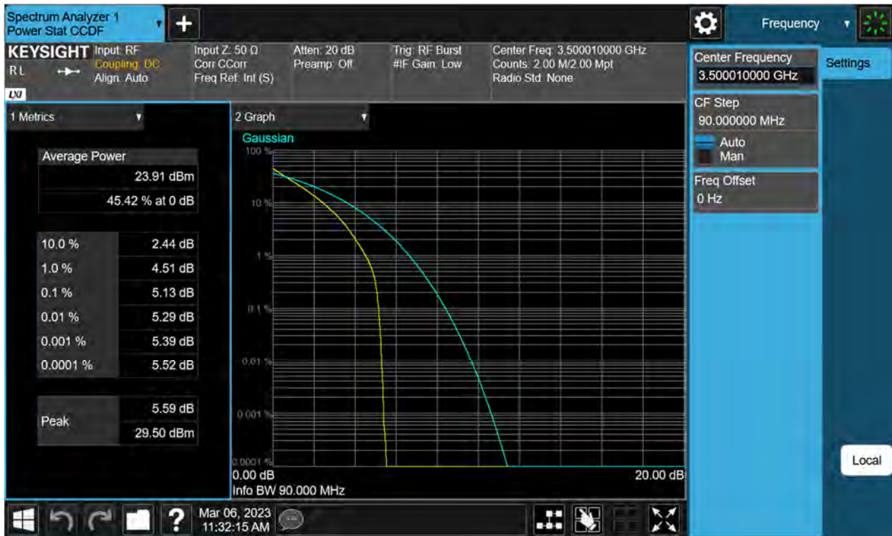
Sub6 n77(78). PAR Plot (90 M BW_Ch.633334_QPSK)
