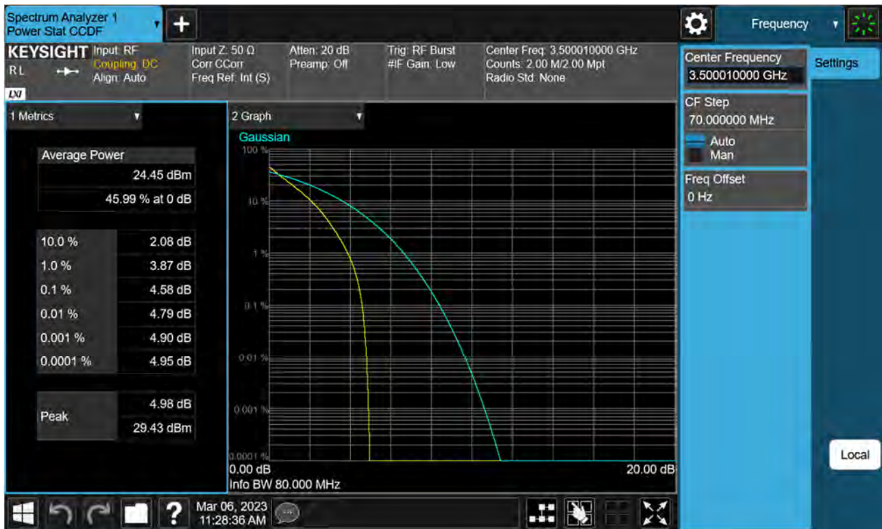
Sub6 n77(78). PAR Plot (80 M BW_Ch.633334_BPSK)
