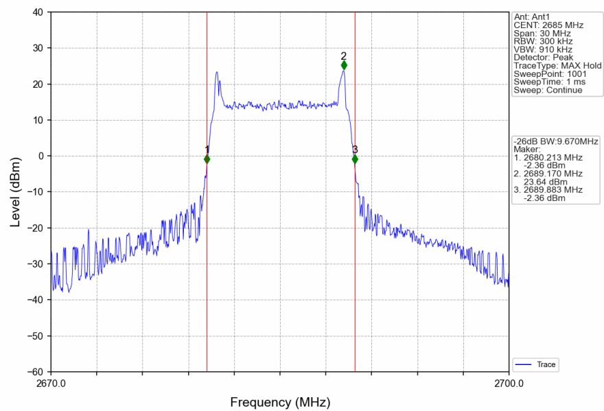
Band41_10MHz_16QAM_HCH_2685MHz_RB_50_0_NTNV
