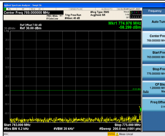
Band13-10MHz-16QAM-23230-1-0-Low-763-775--58.3-PASS
