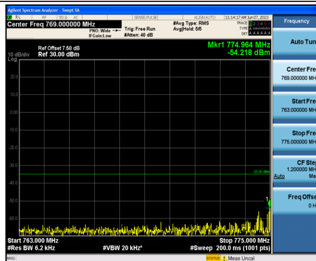
Band13-5MHz-16QAM-23205-1-0-Low-763-775--54.22-PASS
