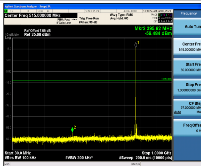
Band13-5MHz-16QAM-23230-1-0-Low-30-1000--59.48-PASS
