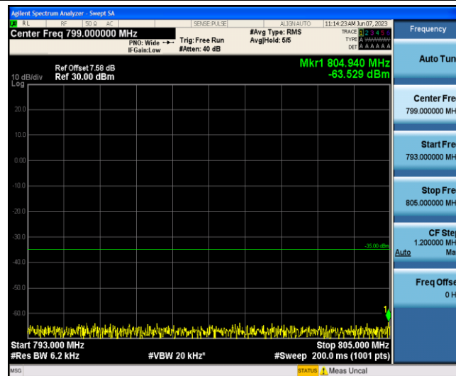
Band13-5MHz-16QAM-23205-1-0-Low-793-805--63.53-PASS
