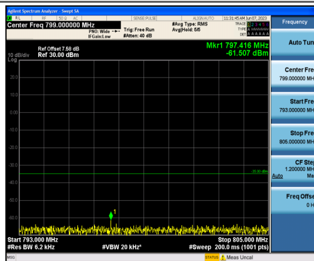
Band13-10MHz-16QAM-23230-1-0-Low-793-805--61.51-PASS
