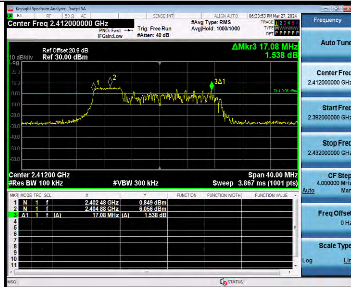
11AX20MIMO_Ant1_2412_106Tone_RU53
