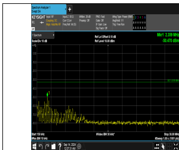
Band66 15MHz 16QAM 132597 1RB#0 0.15~30 0.15~30
