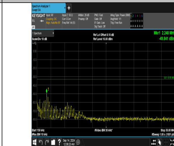
Band66 15MHz QPSK 132597 1RB#74 0.15~30 0.15~30
